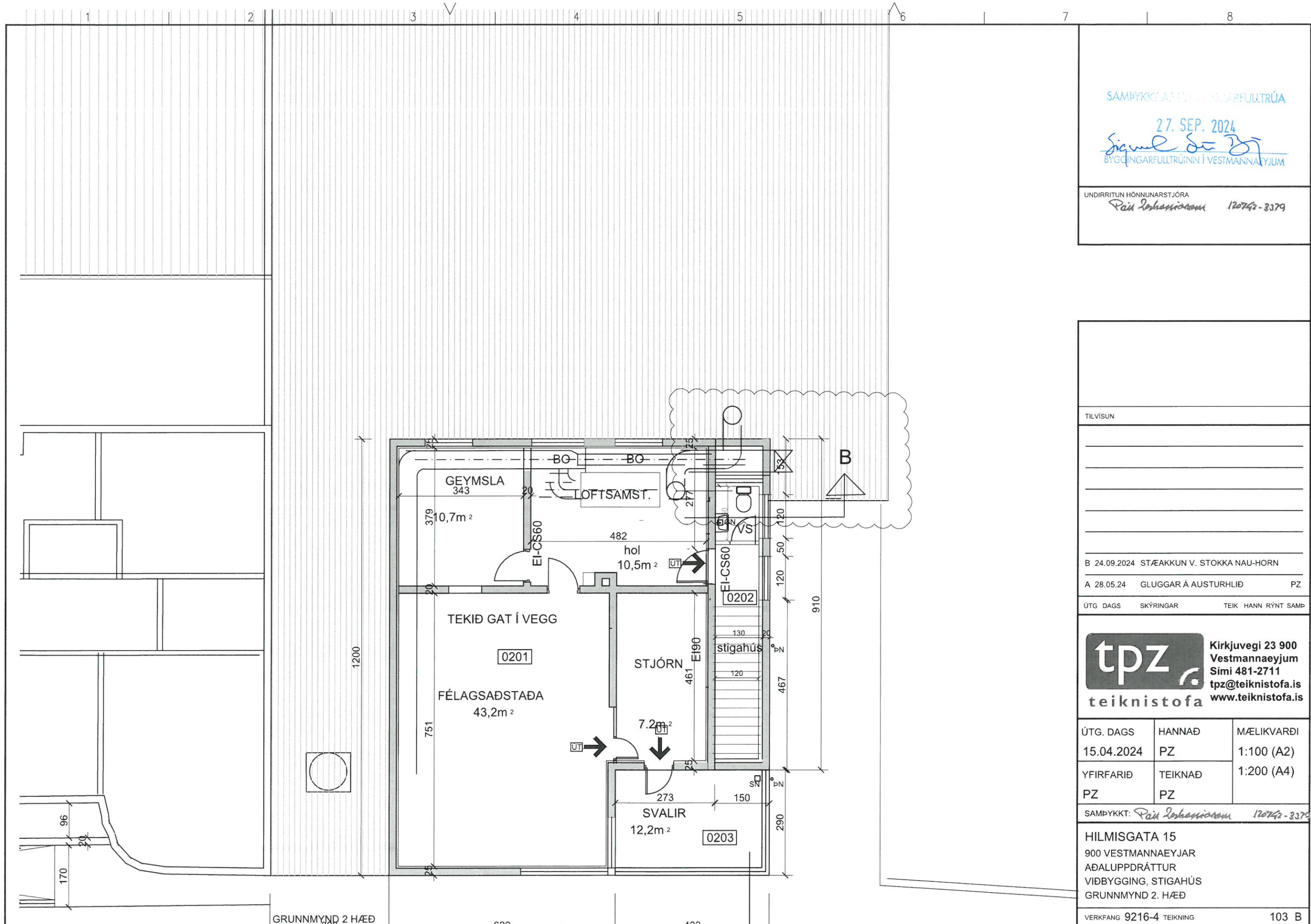
GRUNNMYND 2 HÆÐ
