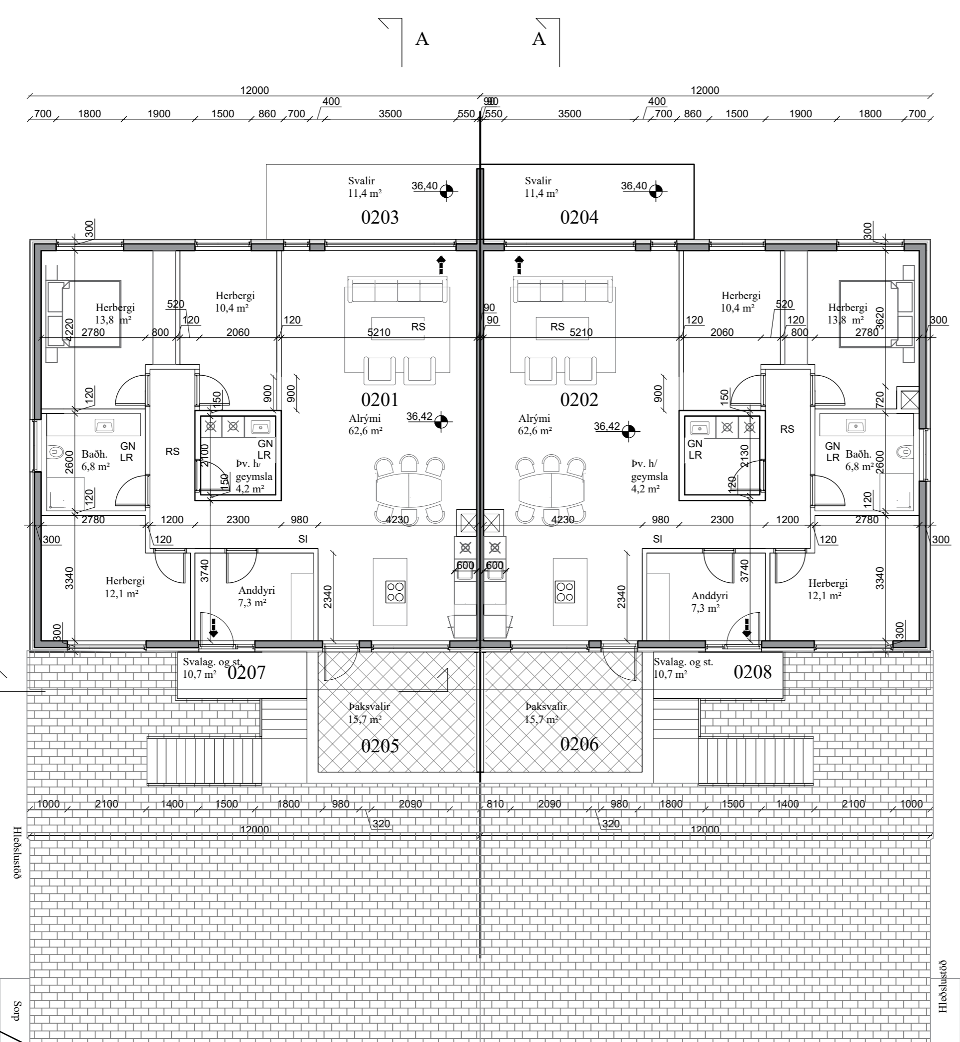
Grunnmynd 2. hæð 1:100
