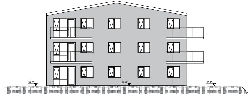
Útlit - vestur 1:100
