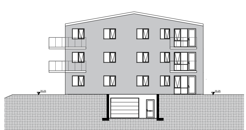
Útlit - austur 1:100
