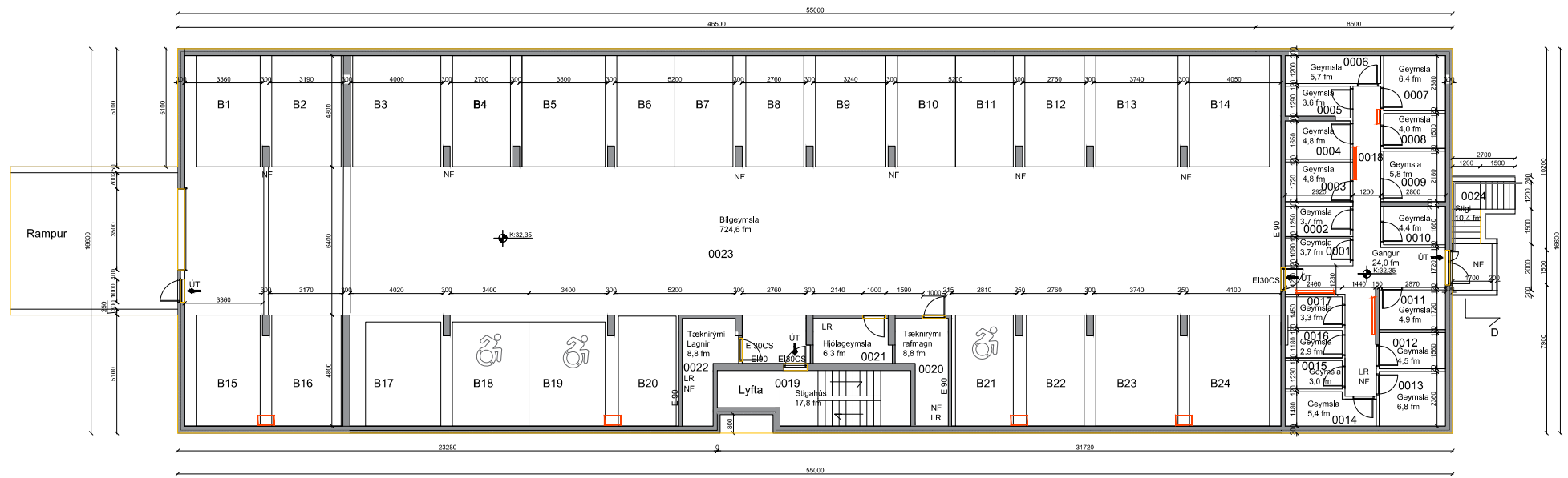
Grunnmynd, kjallari 1:100
