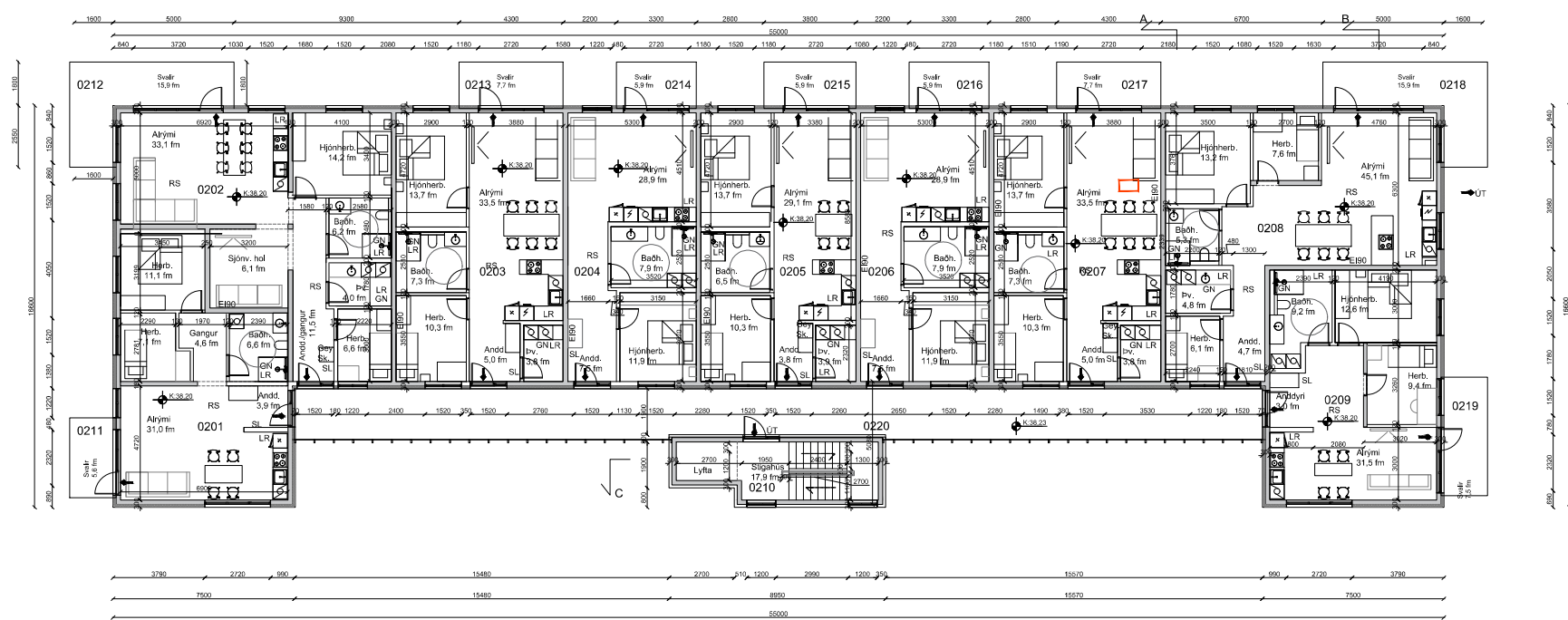
Grunnmynd, 2. hæð 1:100
