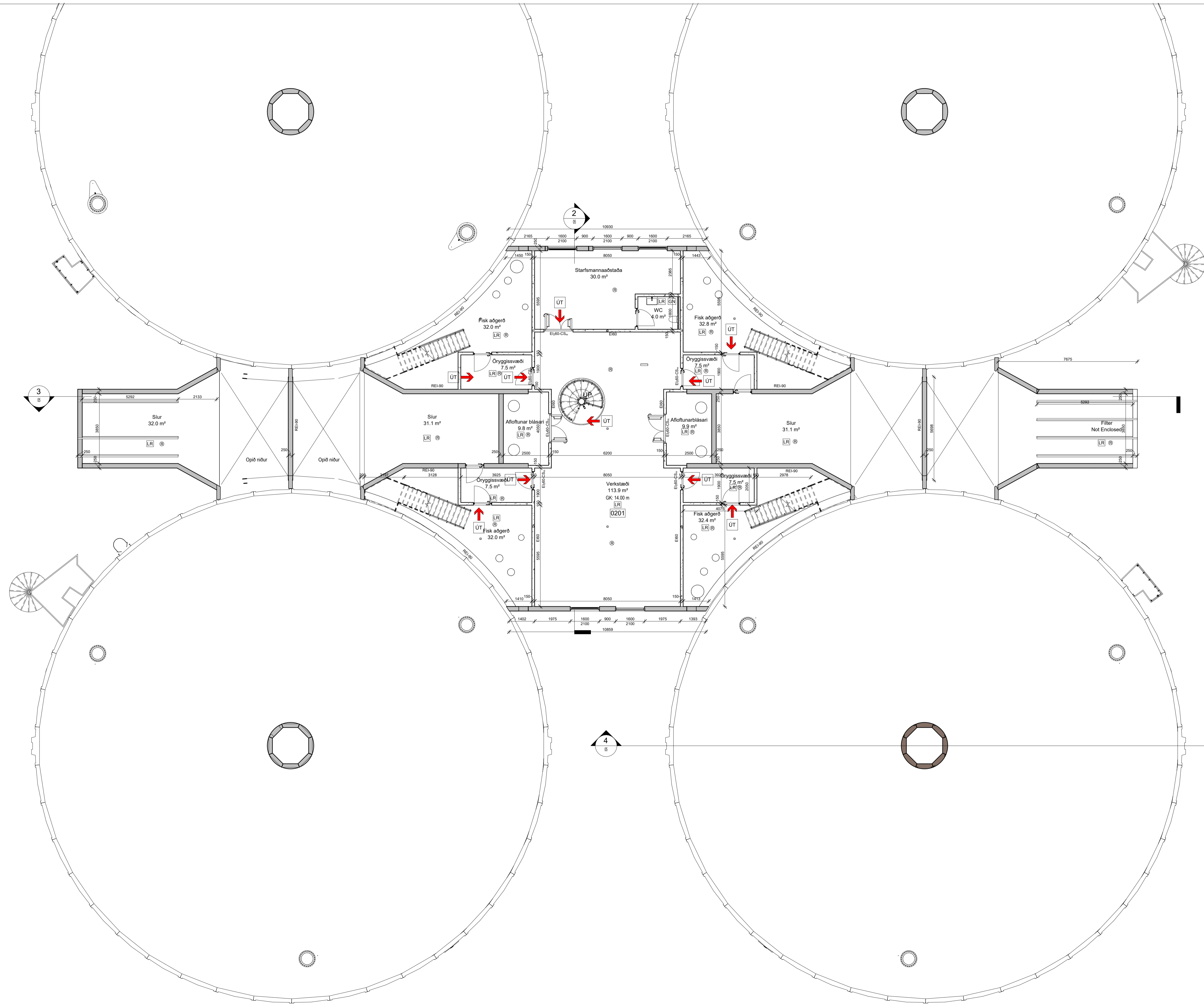
1 Part 11 - 2. hæð Grunnmynd 1 : 100
