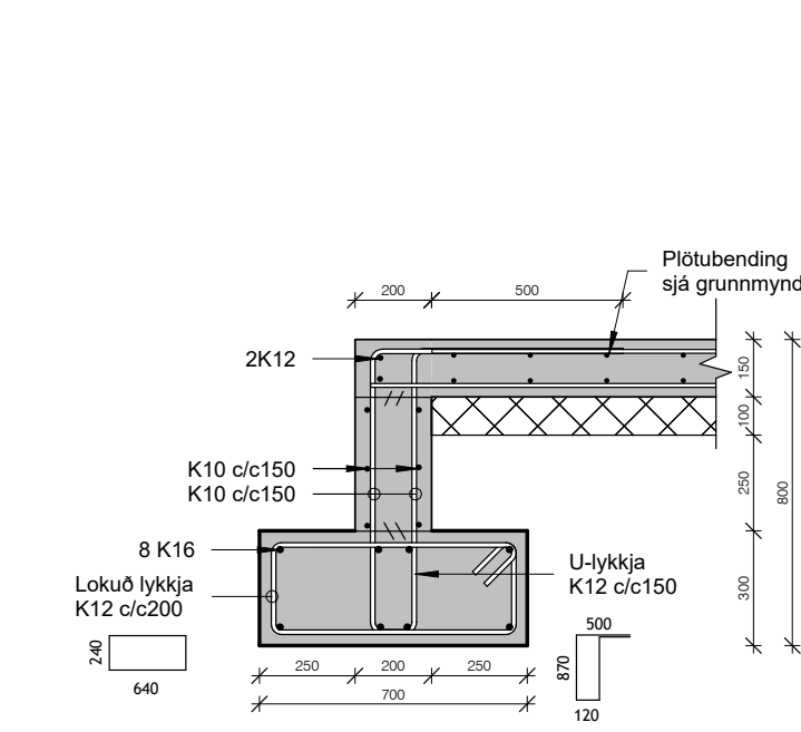
Snið AB 1 : 20
