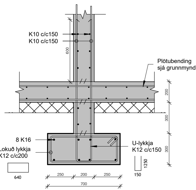
Snið AE 1 : 20
