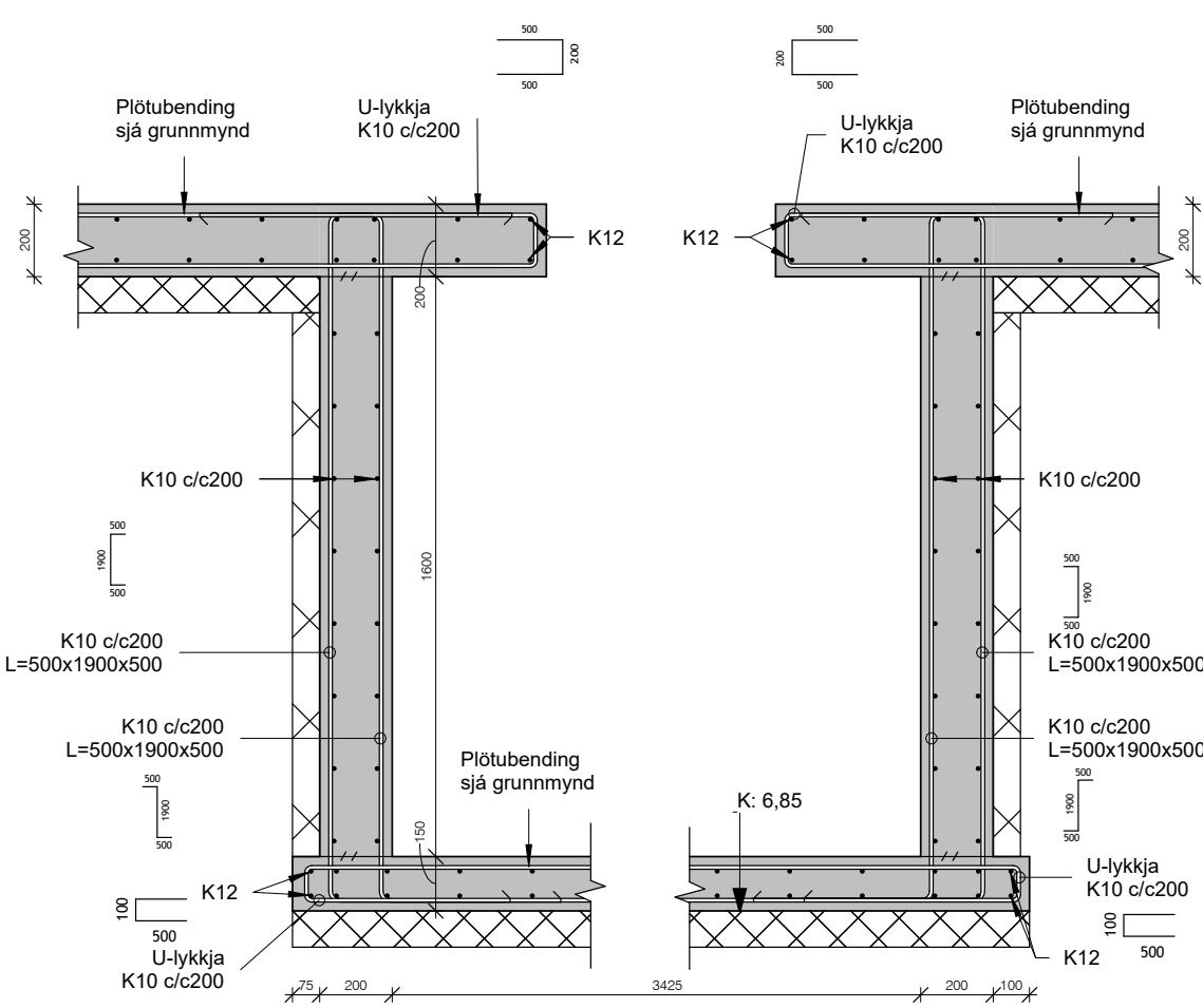
Snið AF 1 : 20
