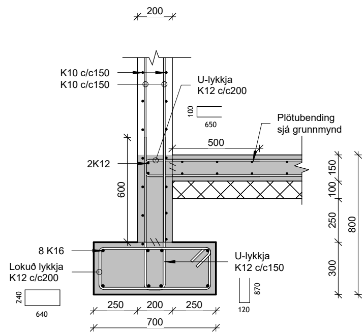
Snið AA 1 : 20
