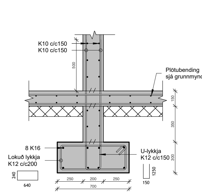
Snið AC 1 : 20
