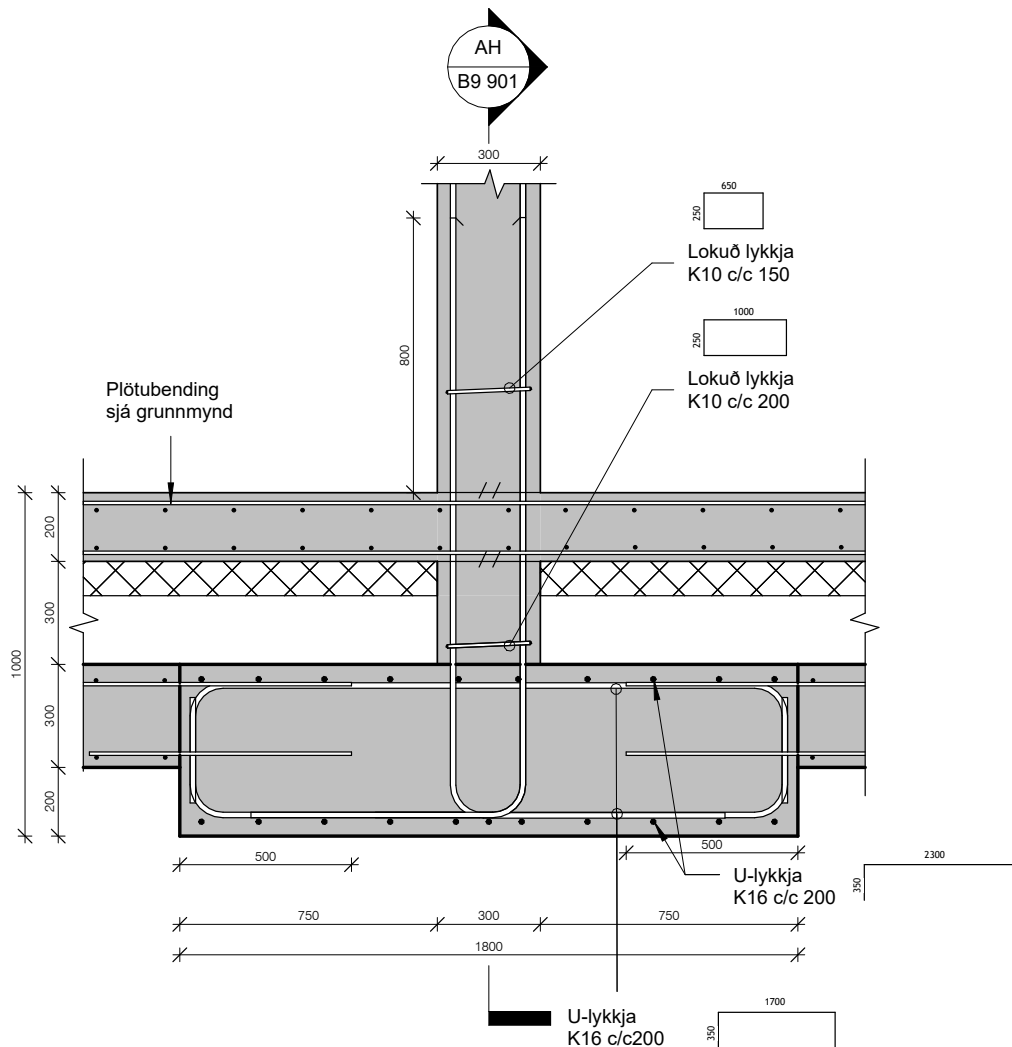
Snið AI 1 : 20
