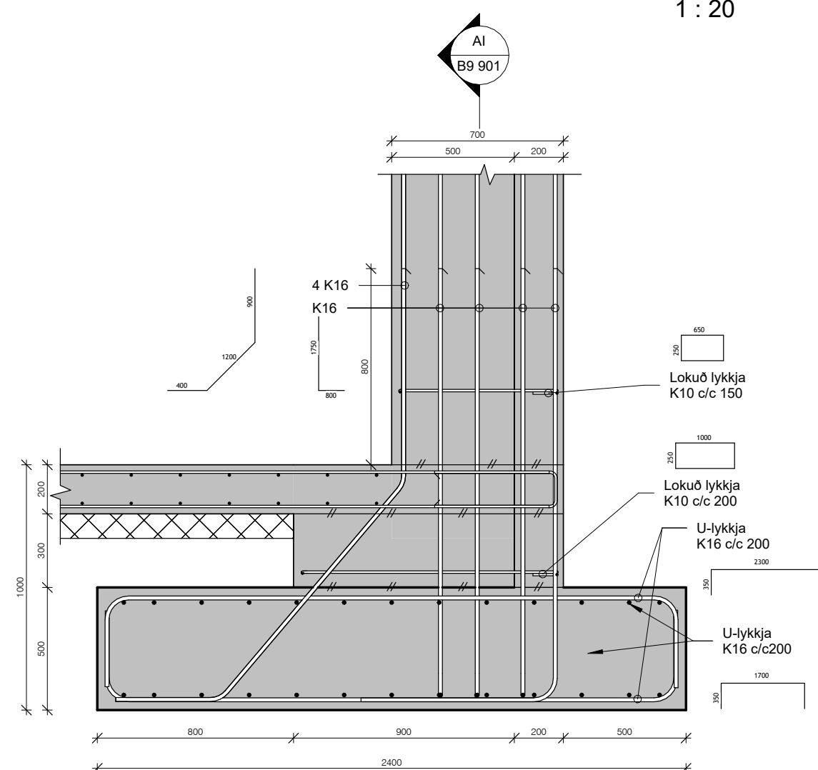
Snið AH 1 : 20
