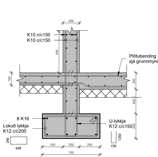
Snið AD 1 : 20
