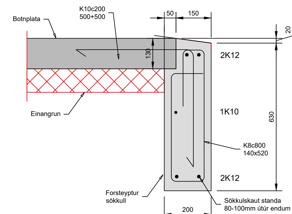
Snið 02 (bílskúrgat)
