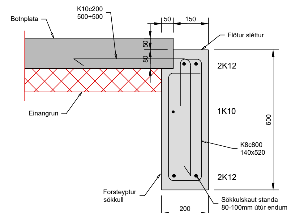
Sniď 01
