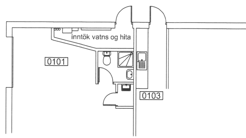
grunnmynd norðausturhluti mkv 1:100
