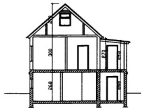
SNID A-A
