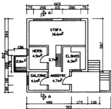
GRUNNMYND HED
