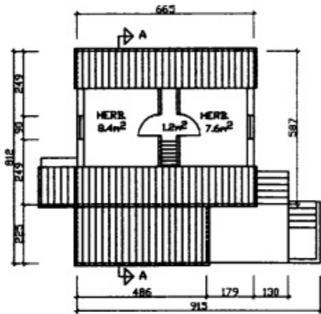
GRUNNMYND RIS
