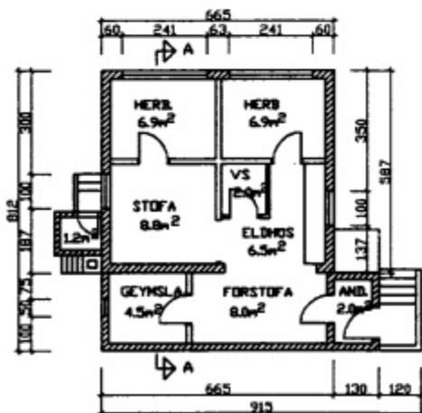
GRUNNMYND KJALLARI
