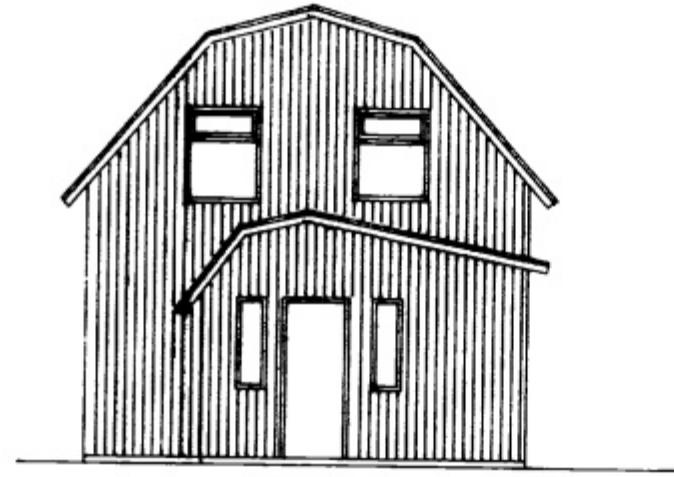
SUÐURHLIÐ Mkv 1:100
