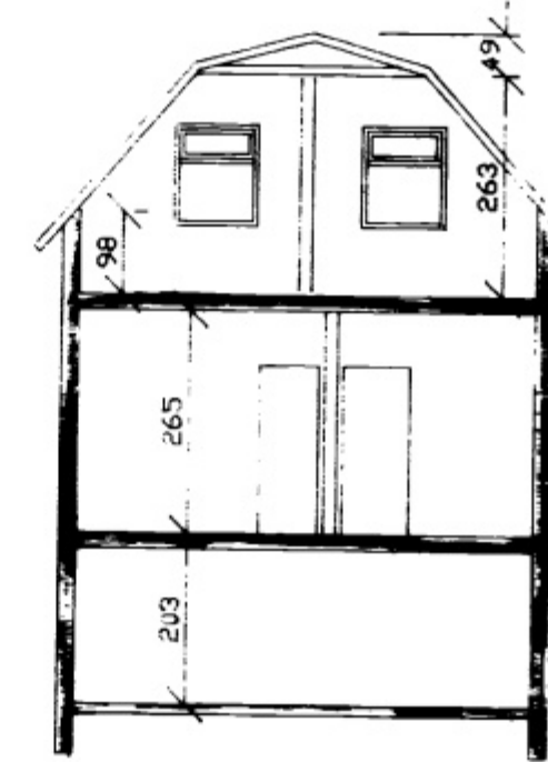
SNIE A-A MKV 1:100
