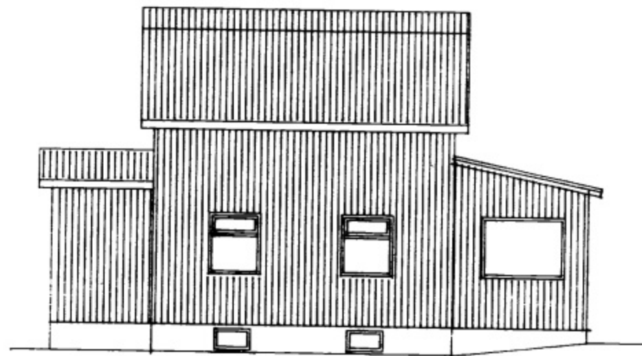
AUSTURHLIÐ Mkv 1:100
