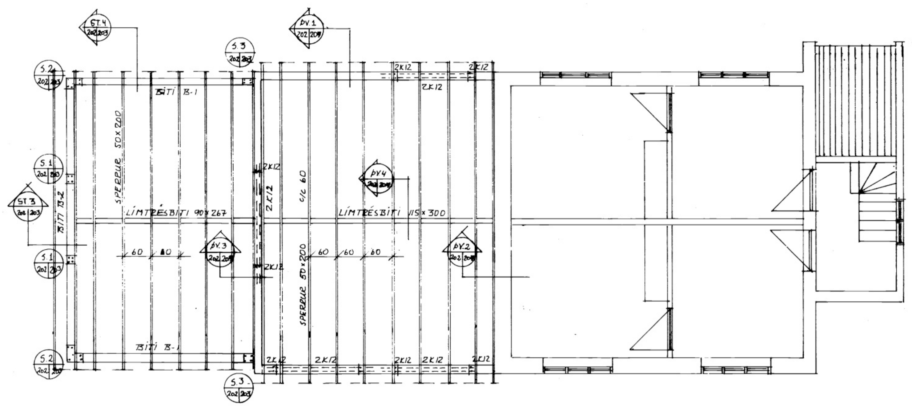
GRUNNMYND AAKYRKA M=1:50
