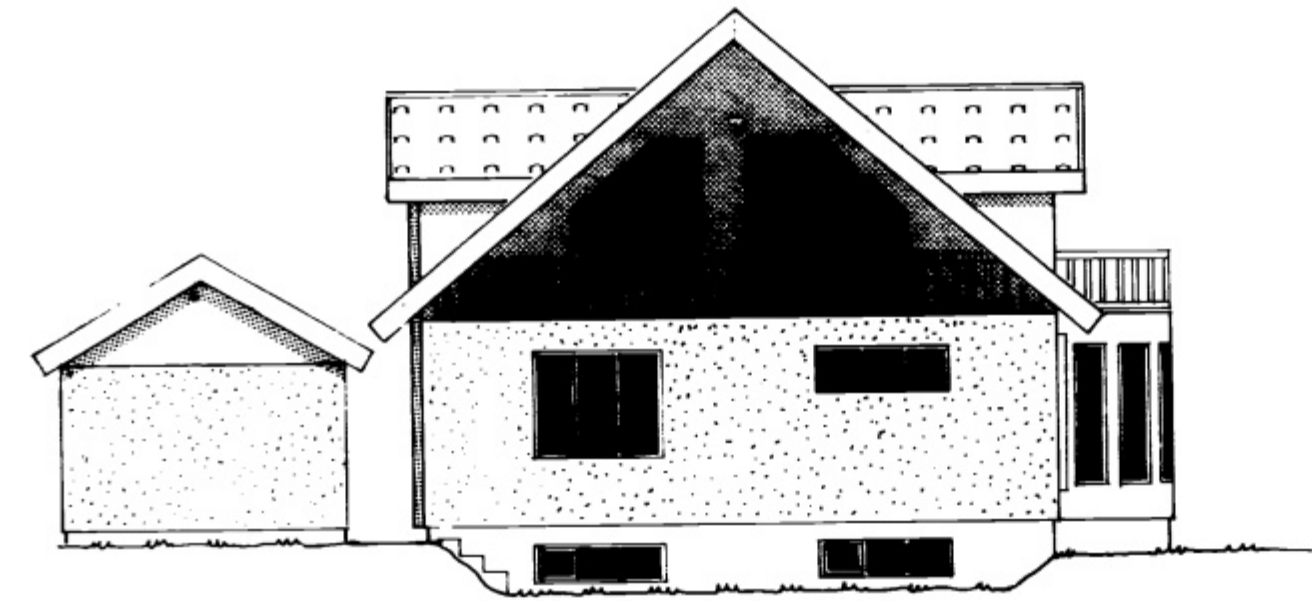
VESTUR 1:100
