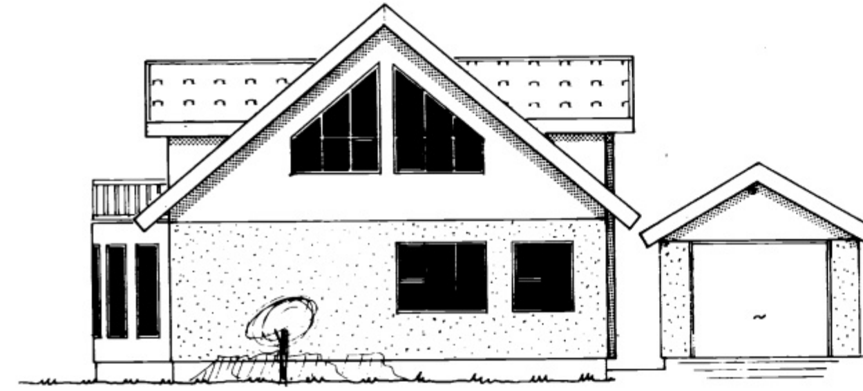
AUSTUR 1:100
