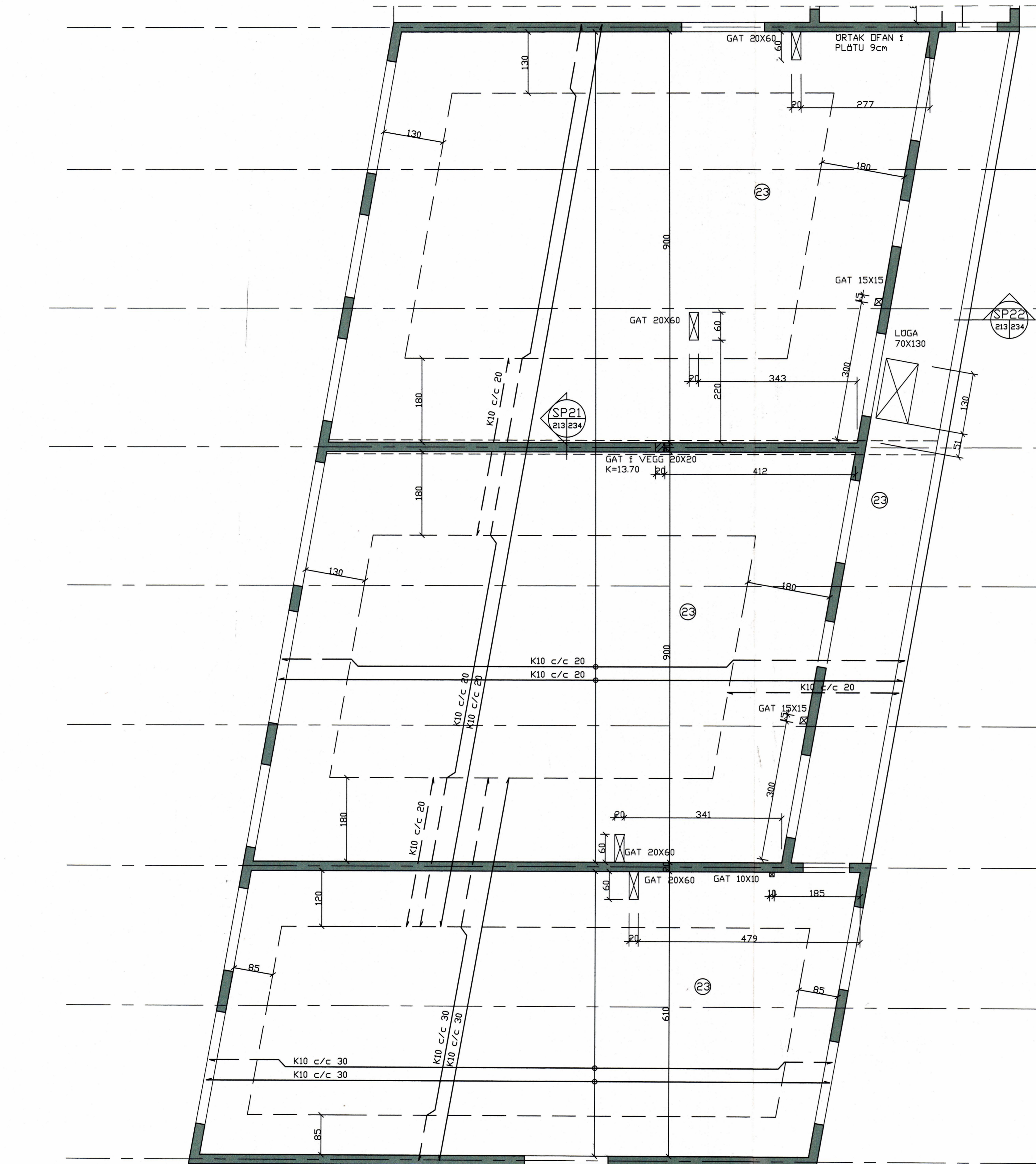
GRUNNMYND PLATA YFIR 3. HÆÐ SUÐURENDI
