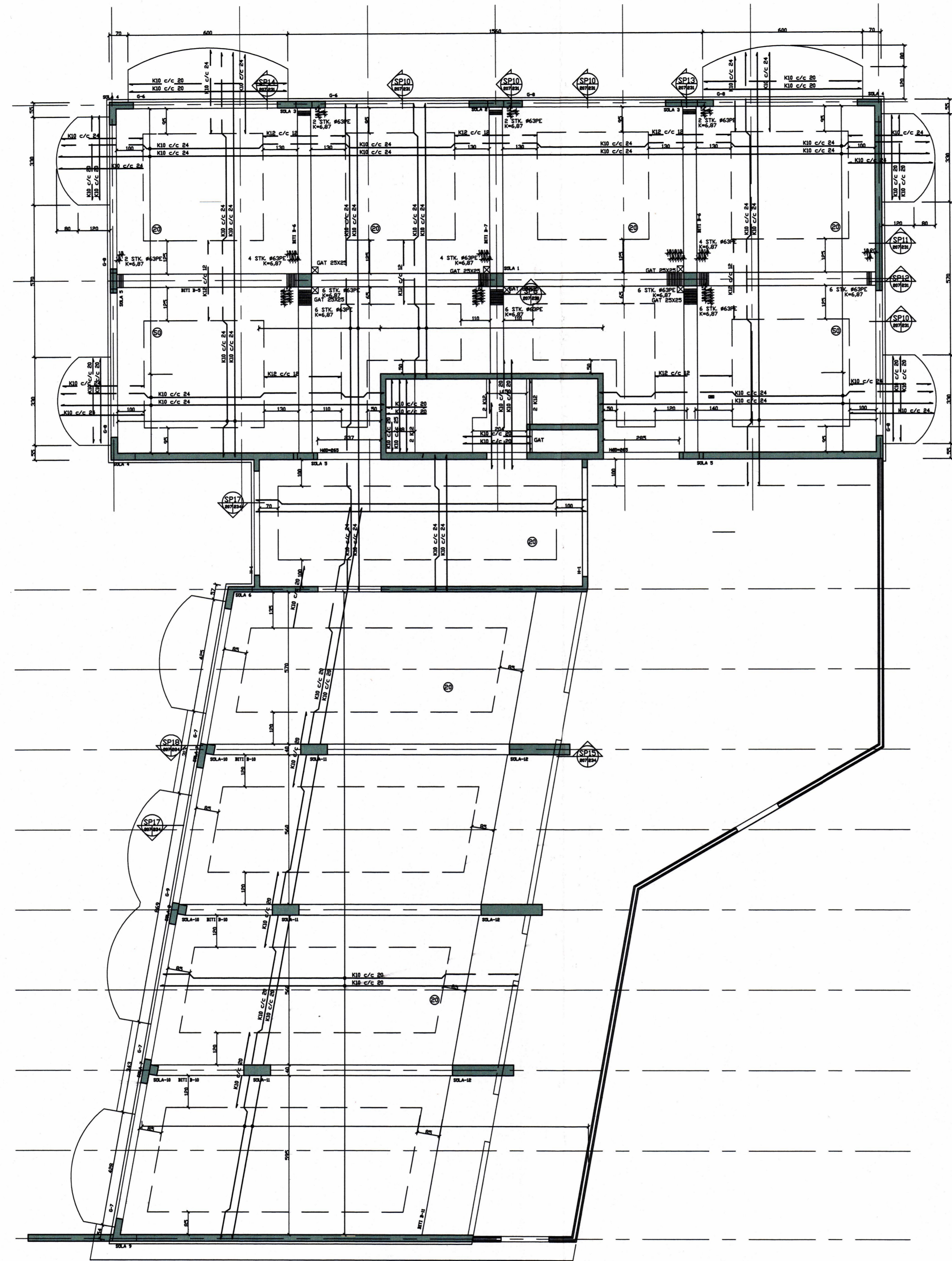
GRUNNMYND PLATA YFIR 1. HÆÐ
