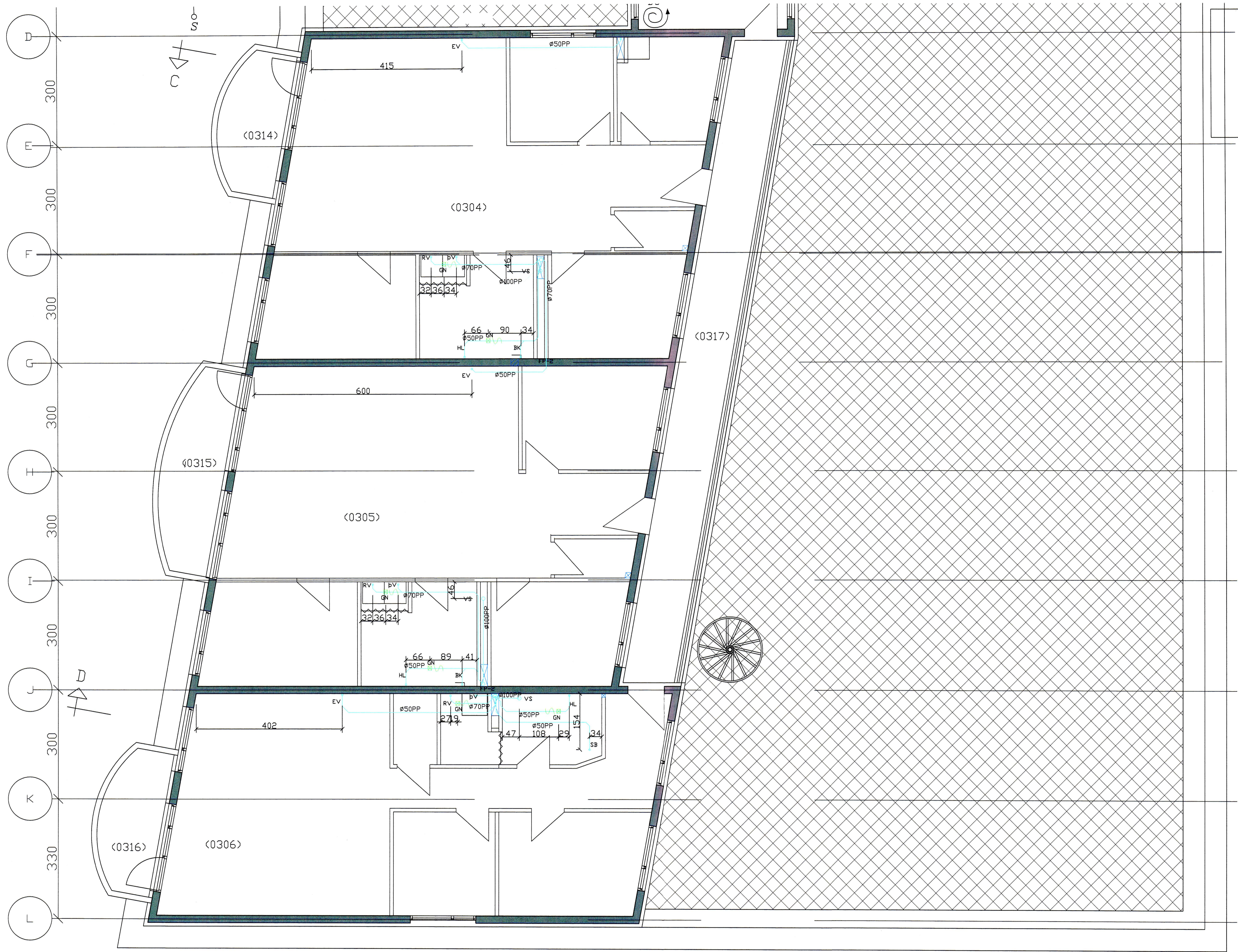
GRUNNMYND 3. HÆÐ
