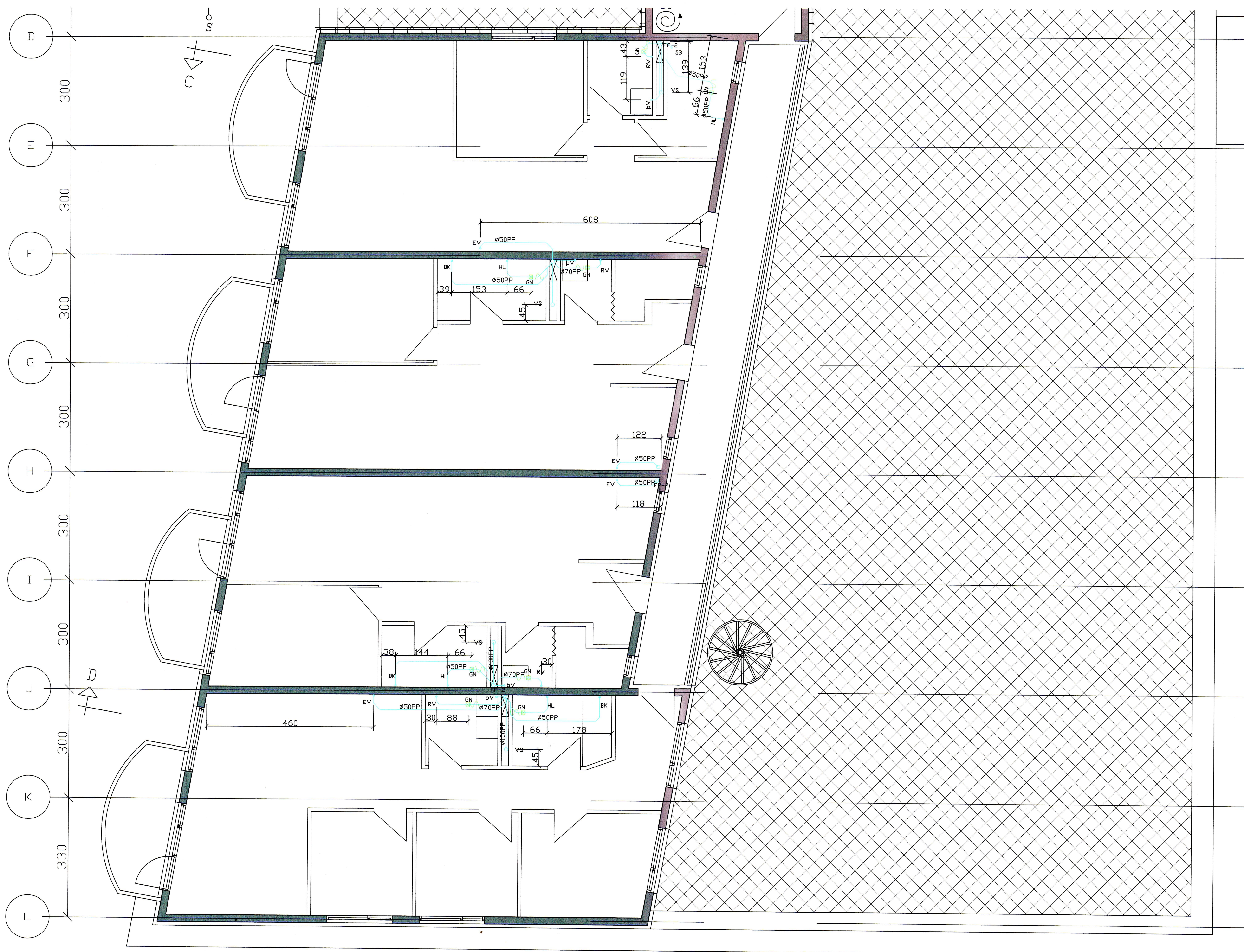
GRUNNMYND 2. HÆÐ
