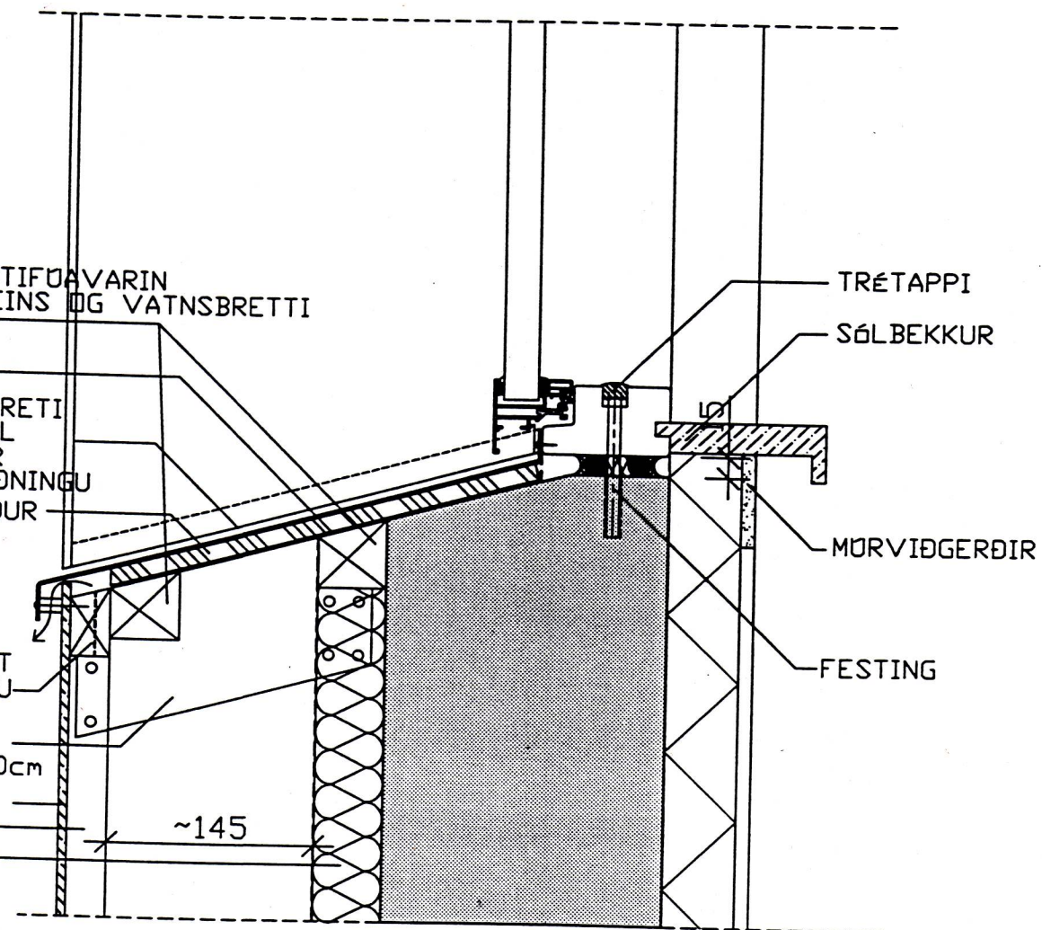
LÓÐRÉTT SNID
