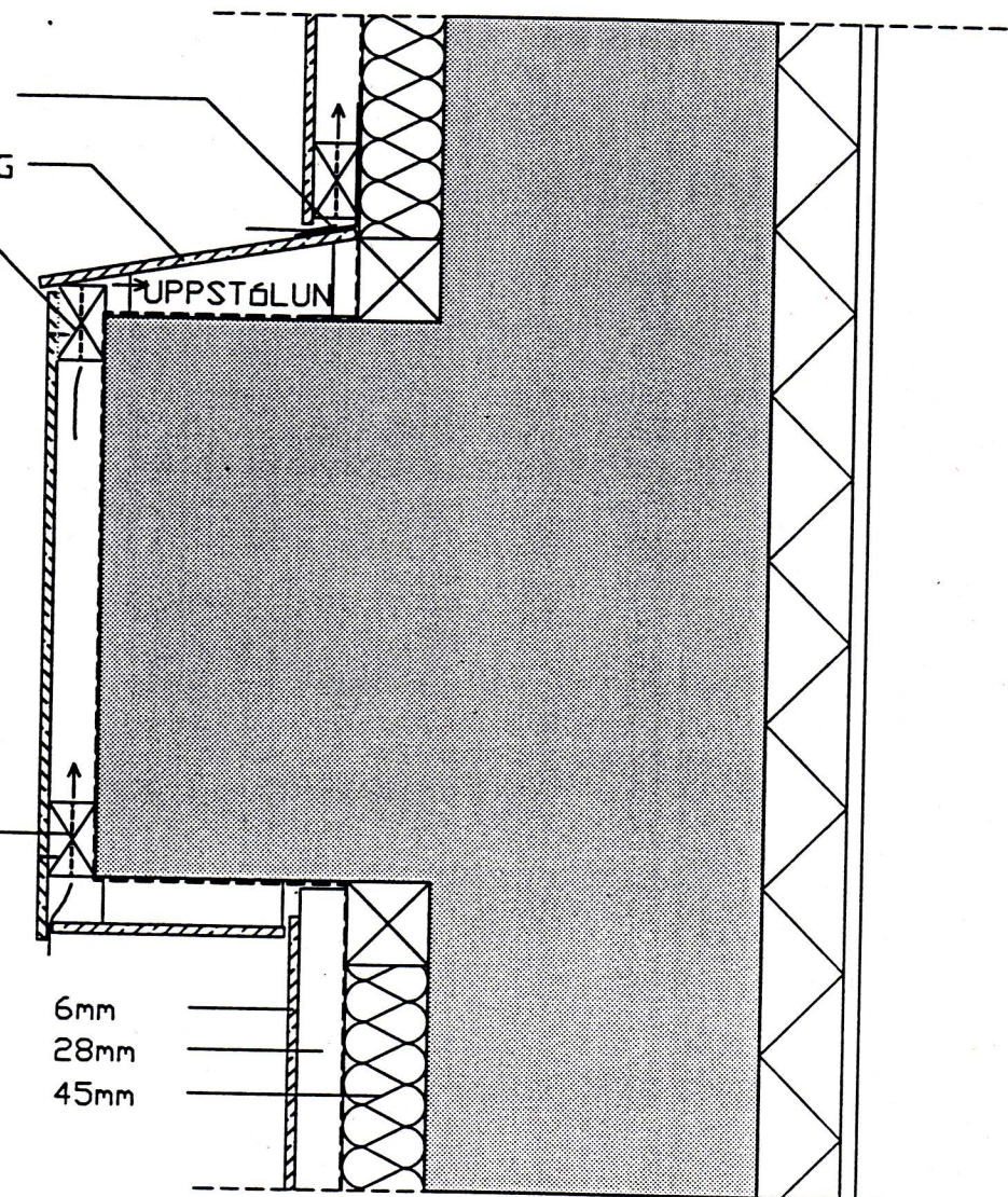
LÓÐRÉTT SNID
