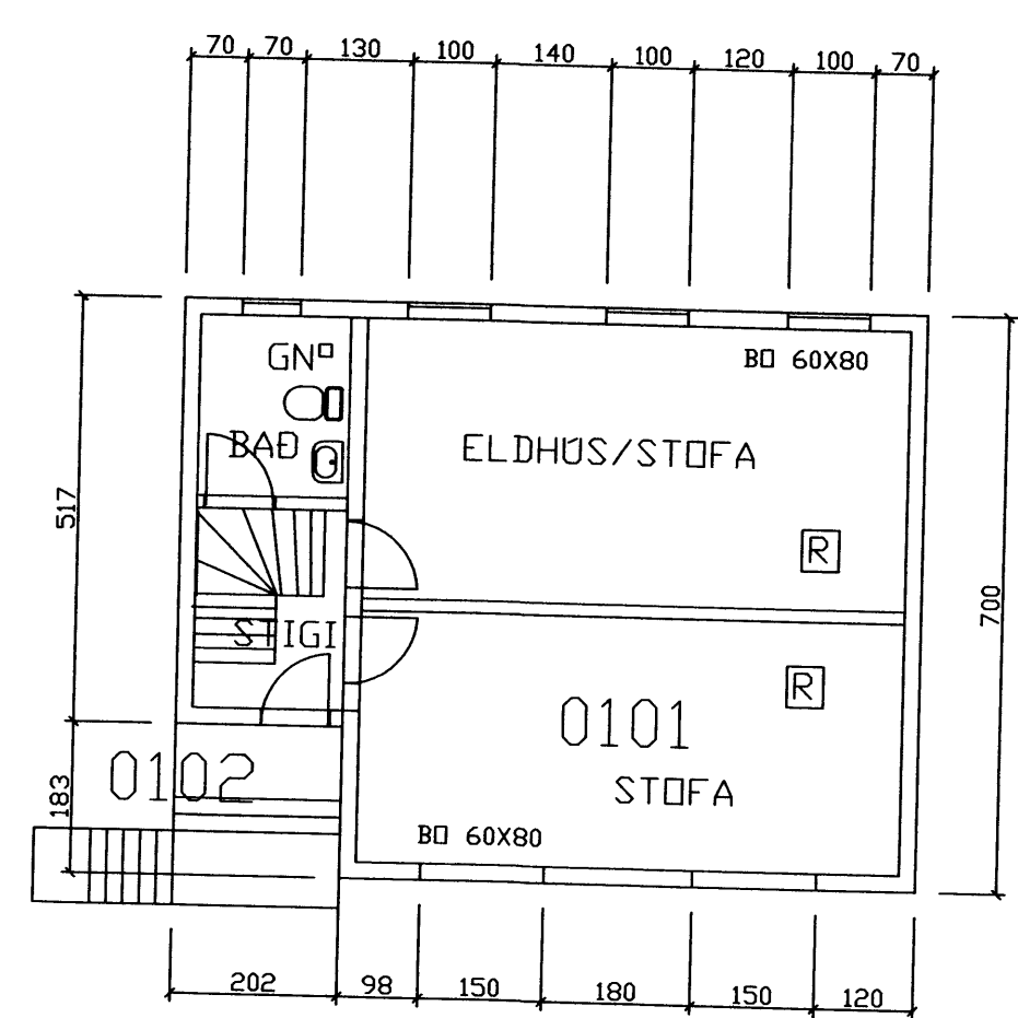
1. HÆÐ
