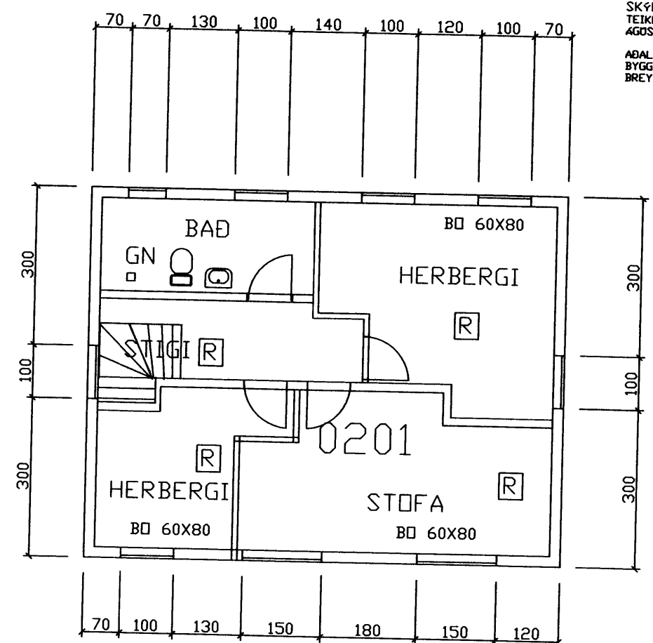
2. HÆÐA/ RIS
