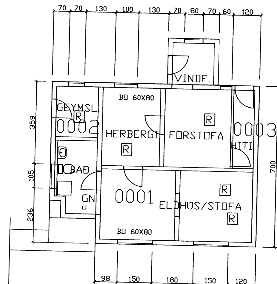
KJALLARI
