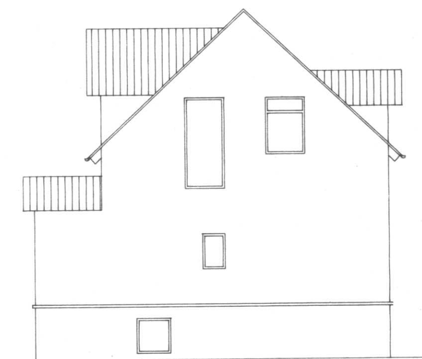
AUSTURHLID M=1:100
