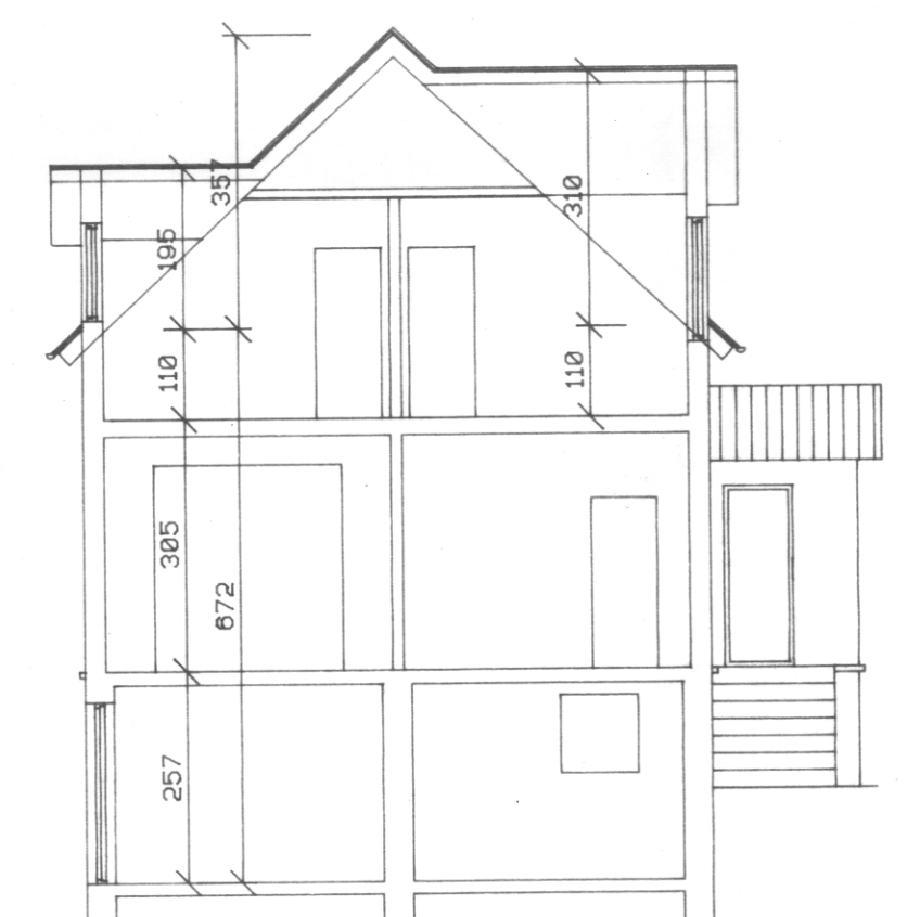
SNIÐ M=1:100
