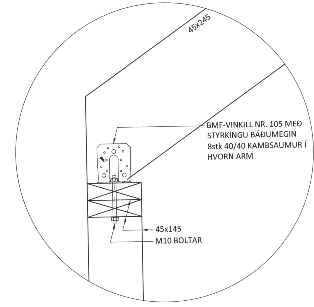
SME 07 M 1:5
