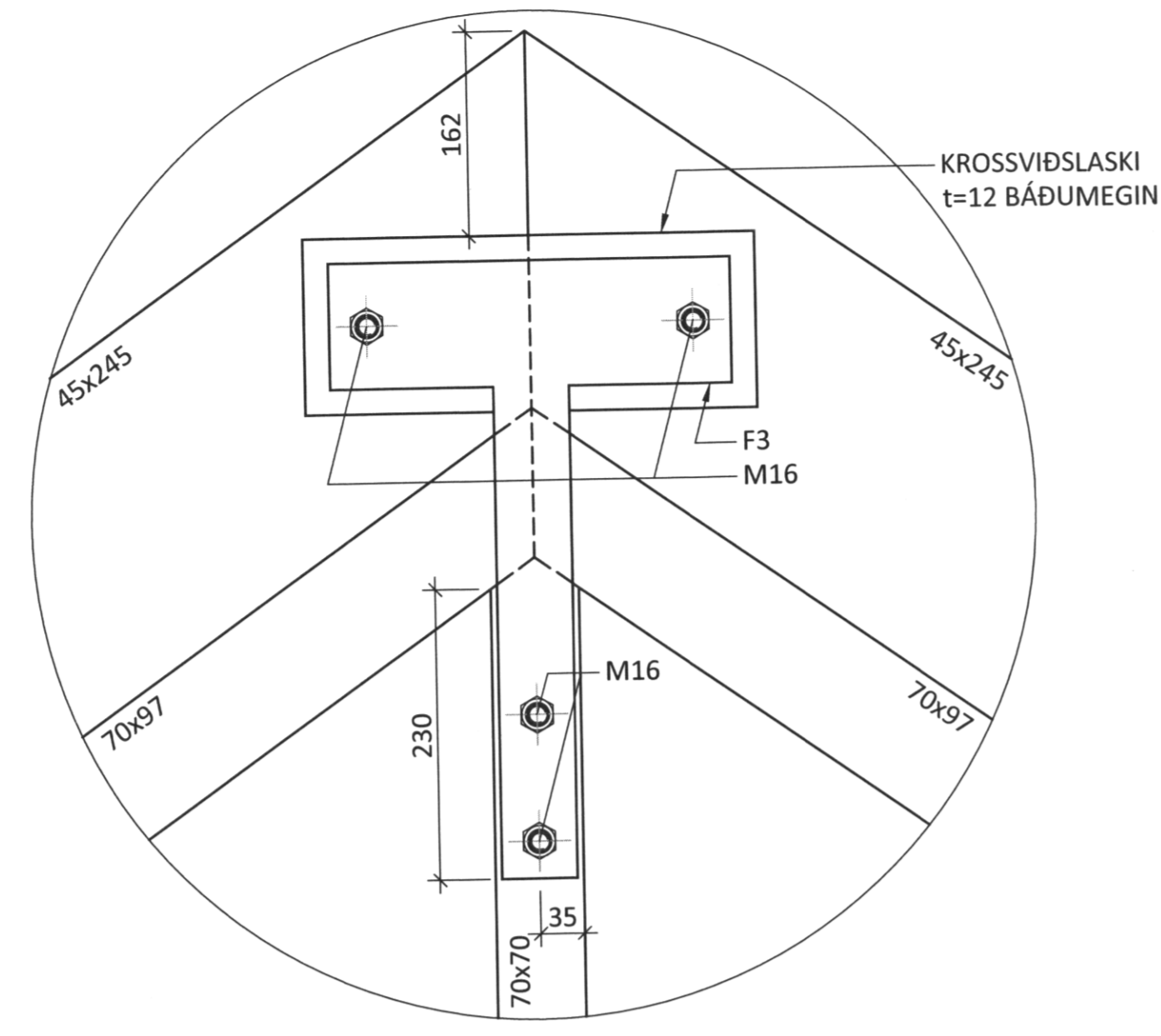
SME 07 M 1:5
