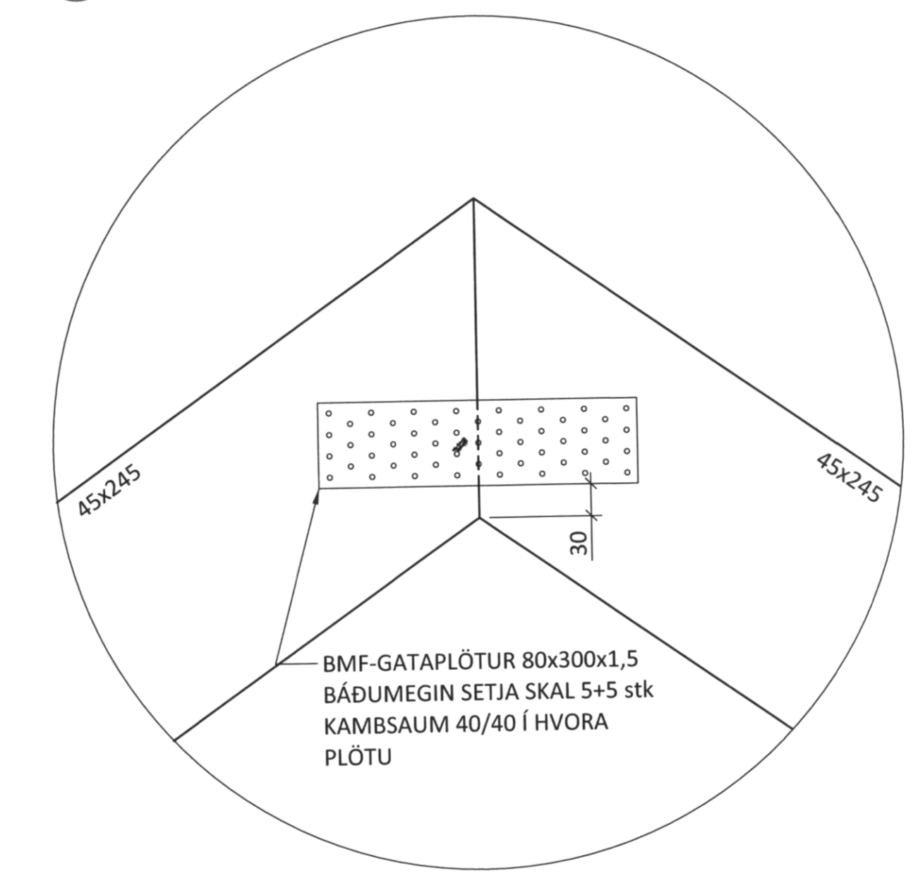
SMF 07 M 1:5
