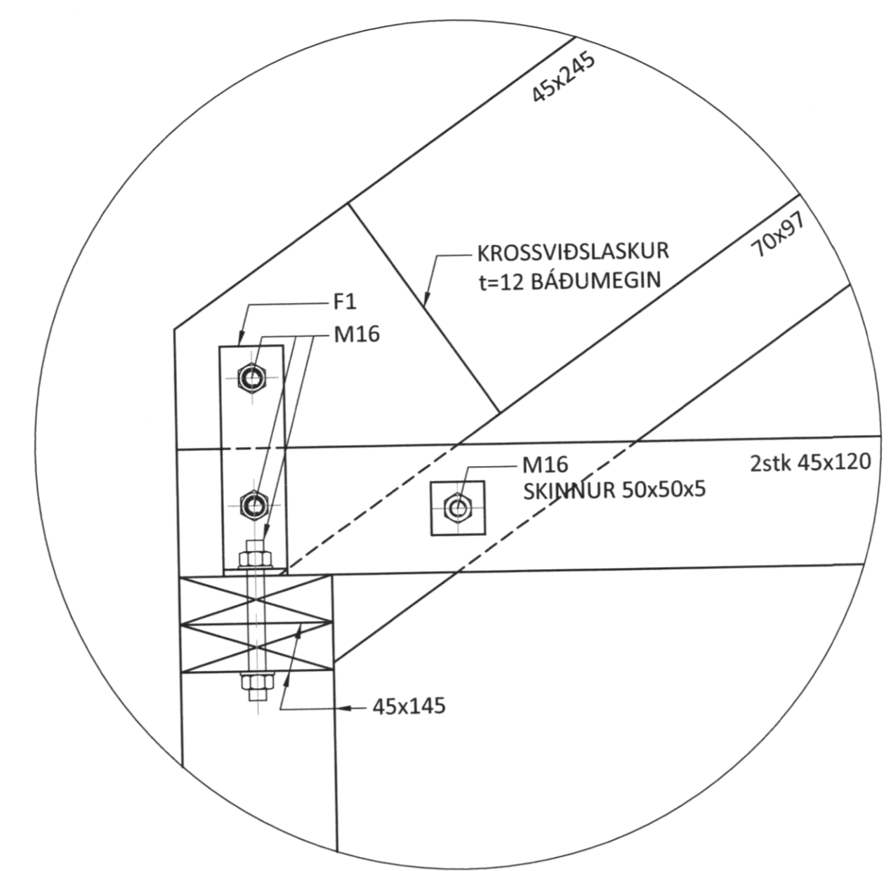
SMF 07 M 1:5
