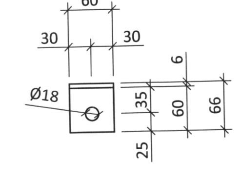
SNÍÐ X - X M1:5
