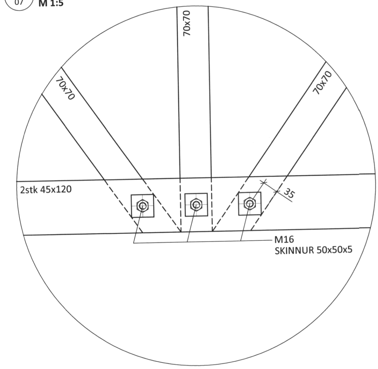
FESTING F1 M1:5
