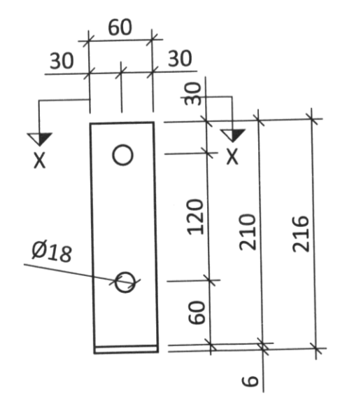
SNÍÐ X - X M1:5
