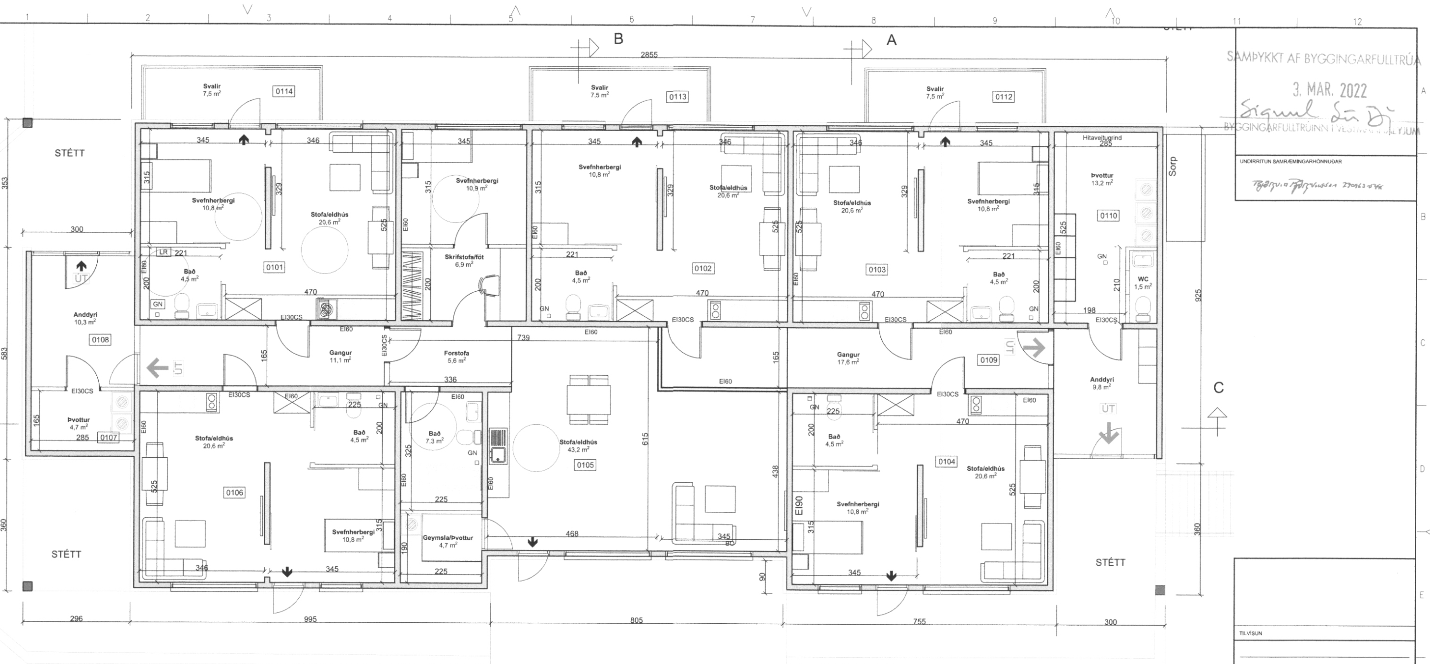
GRUNNMYND, 1. HÆÐ 1:50
