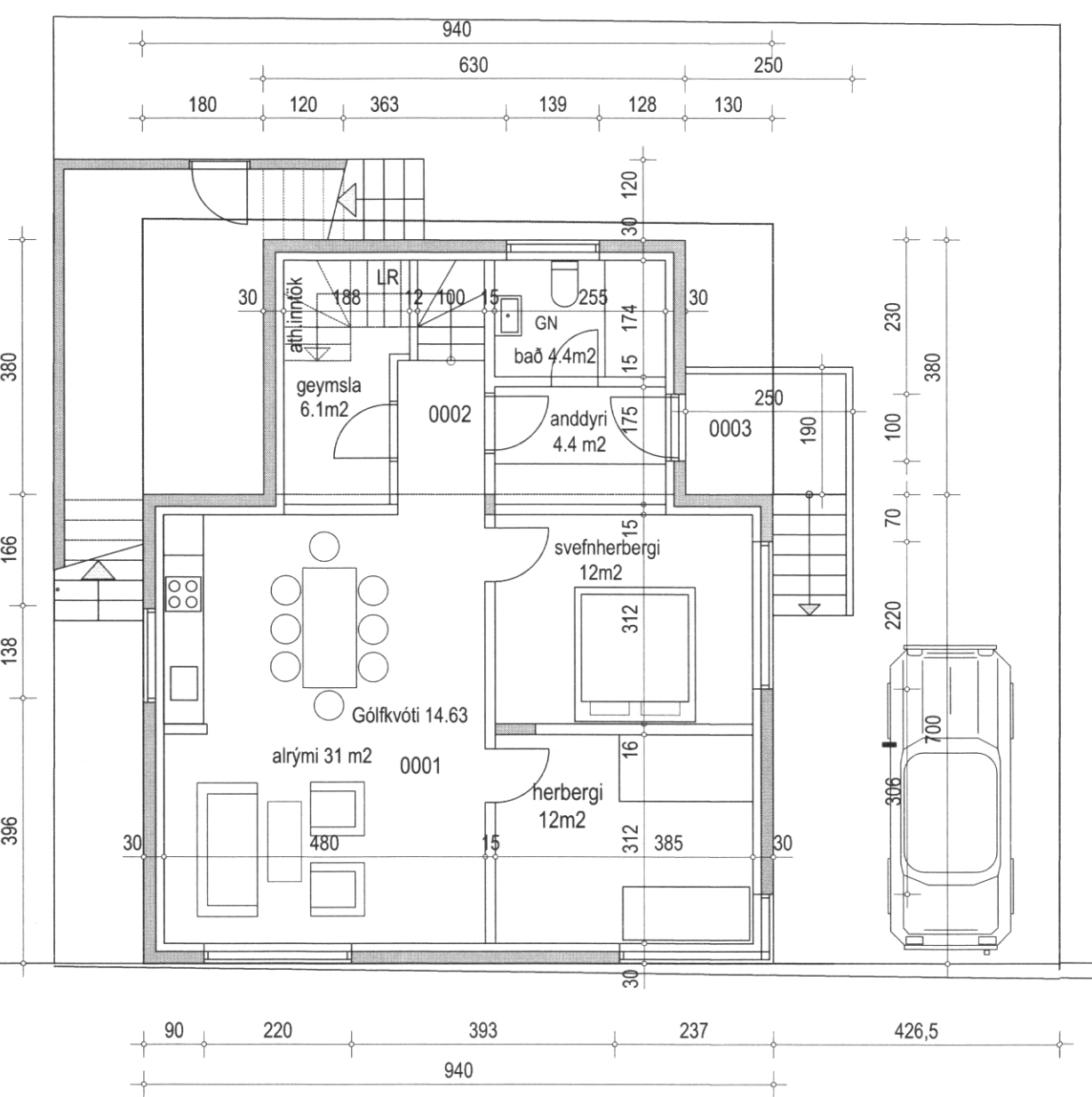
Grunnmynd kjallari mkv 1:100
