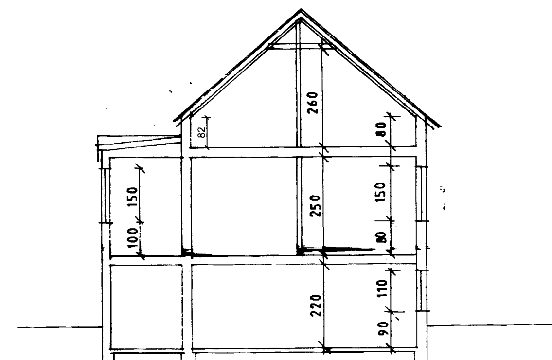
PVERSNID Mkv. 1:100
