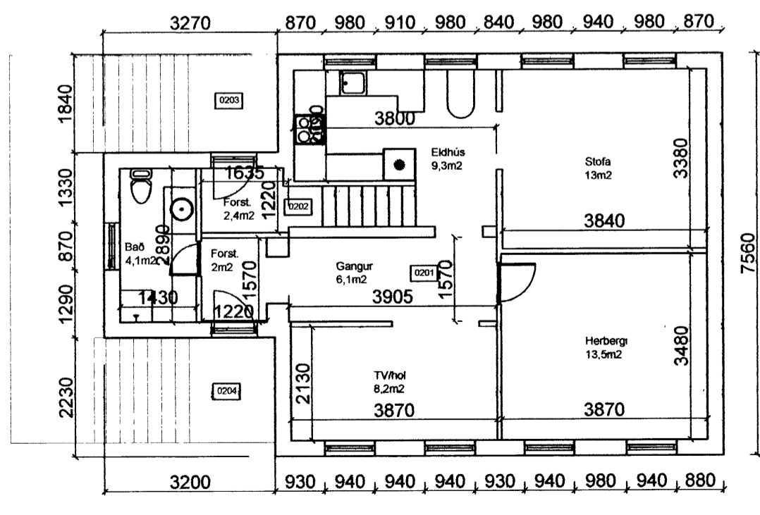
2.HÆÐ
