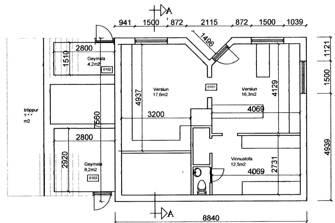
1.HÆÐ
