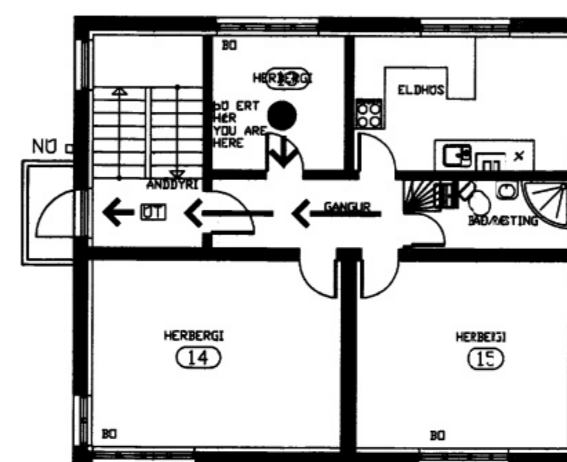
GRUNNMYND 2. HÆÐ
