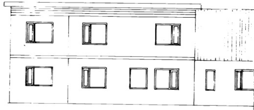
NORÐURHLIÐ MKV 1:100
