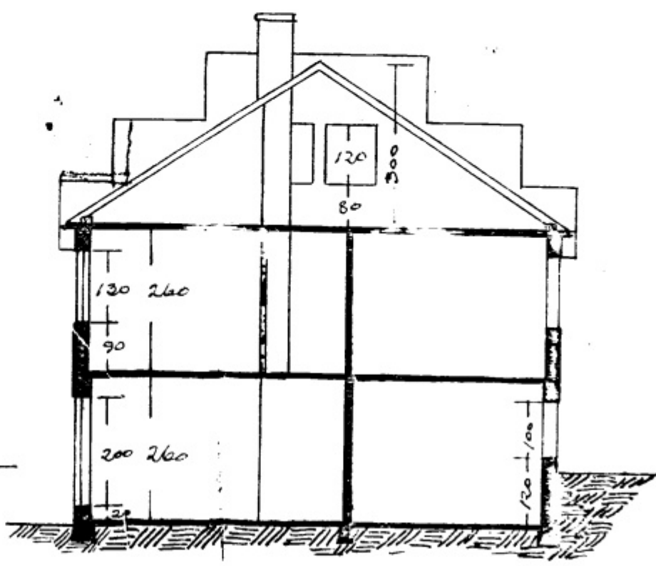
SKURÐUR
