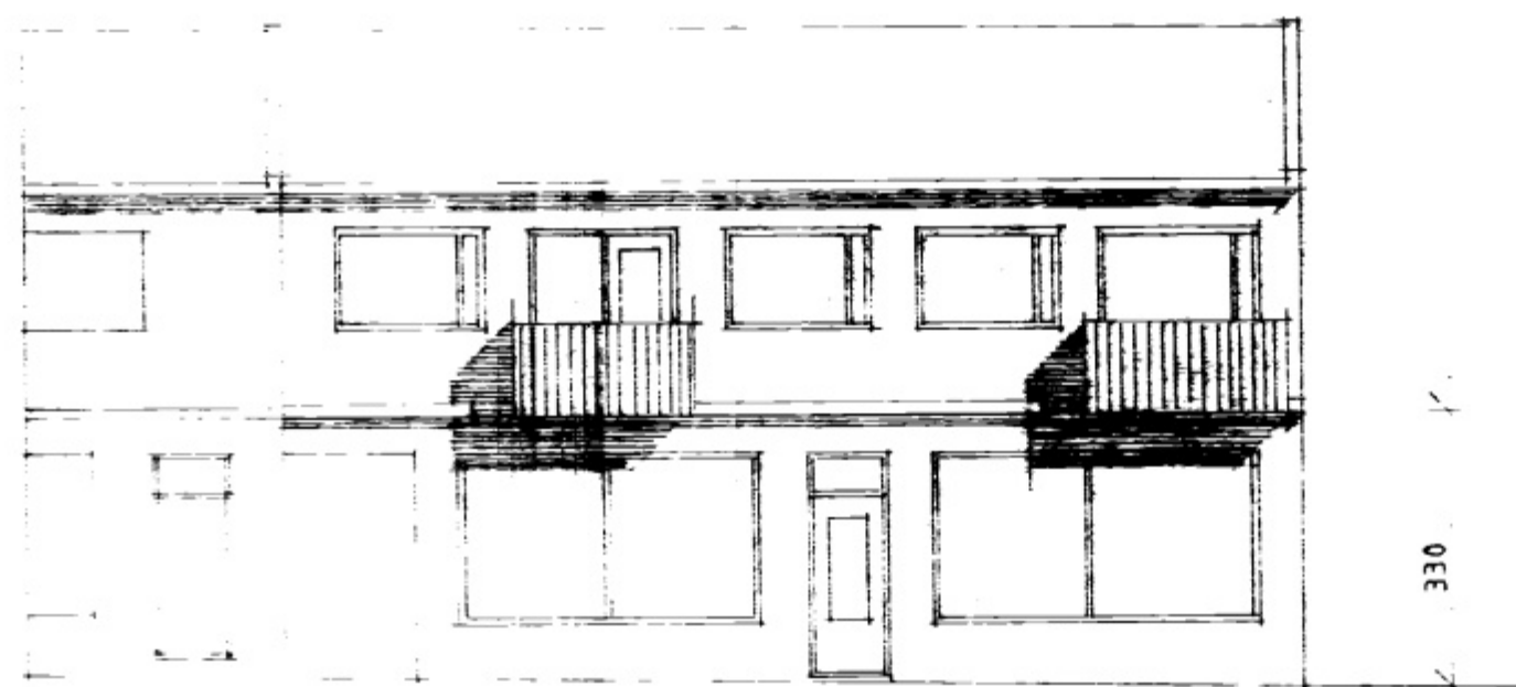
SUÐURHLIÐ
