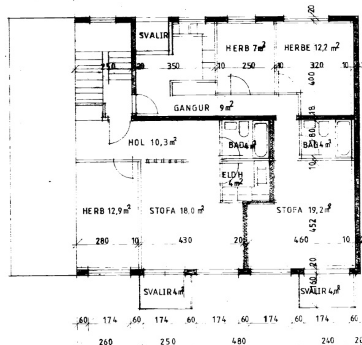
GRUNNMYND 2 HÆÐ 1:100
