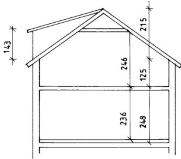
SNID D-D
