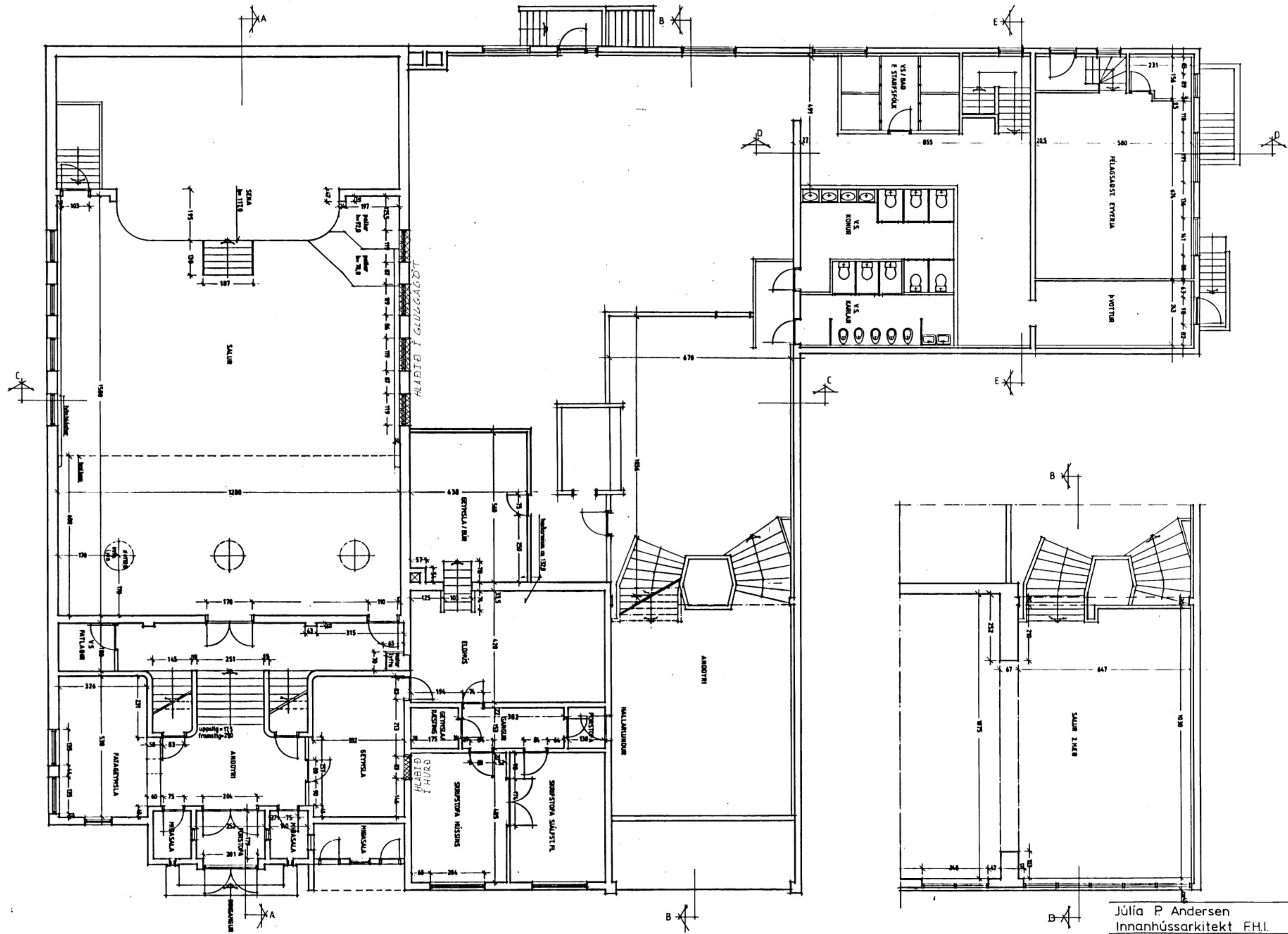
GRUNNMYND 1. HÆÐAR, MKV. 1:100, UPPMÆLING.
