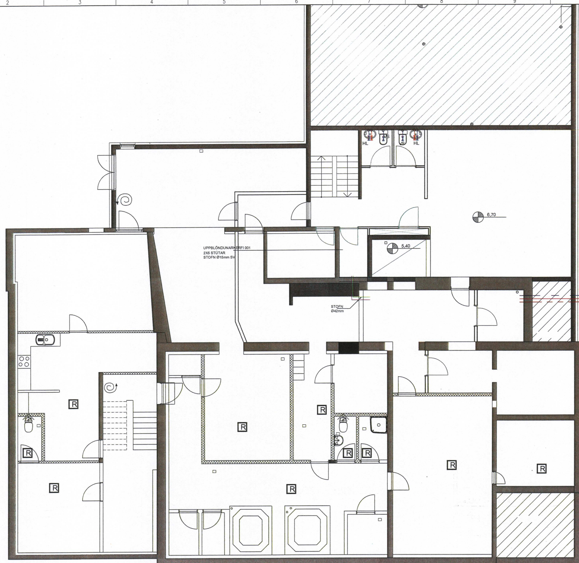
GRUNNMYND KJALLARI VATNSLAGNIR M=1:50
