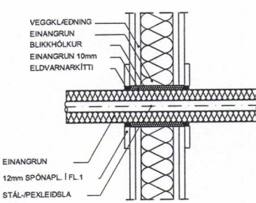
FRÁGANGUR Á STÁL-/PEXLEIÐSLU GEGNUM LÉTTAN VEGG
