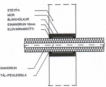
FRÁGANGUR Á STÁL-/PEXLEIÐSLU GEGNUM STEYPTAN VEGG
