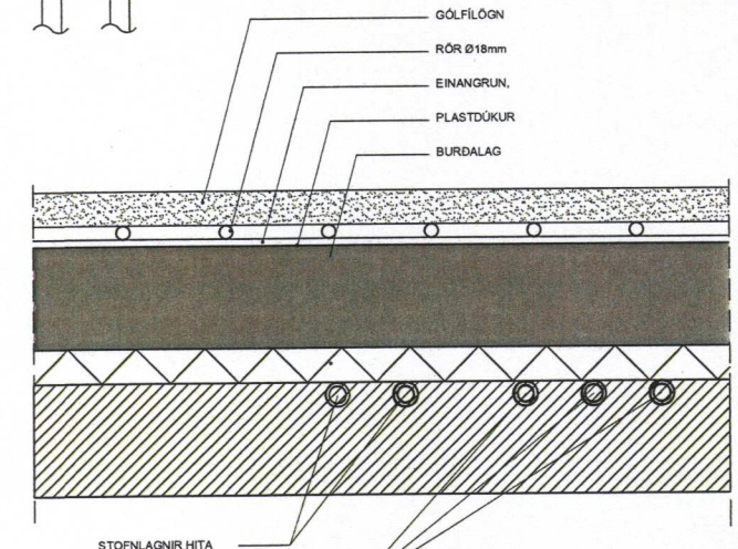
FRÁGANGUR LAGNA Í GÓLF
