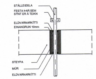
FRÁGANGUR Á STÁLLEIÐSLU GEGNUM STEYPT GÓLF
