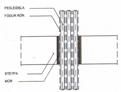
FRÁGANGUR Á PEXLEIÐSLU GEGNUM STEYPT GÓLF
