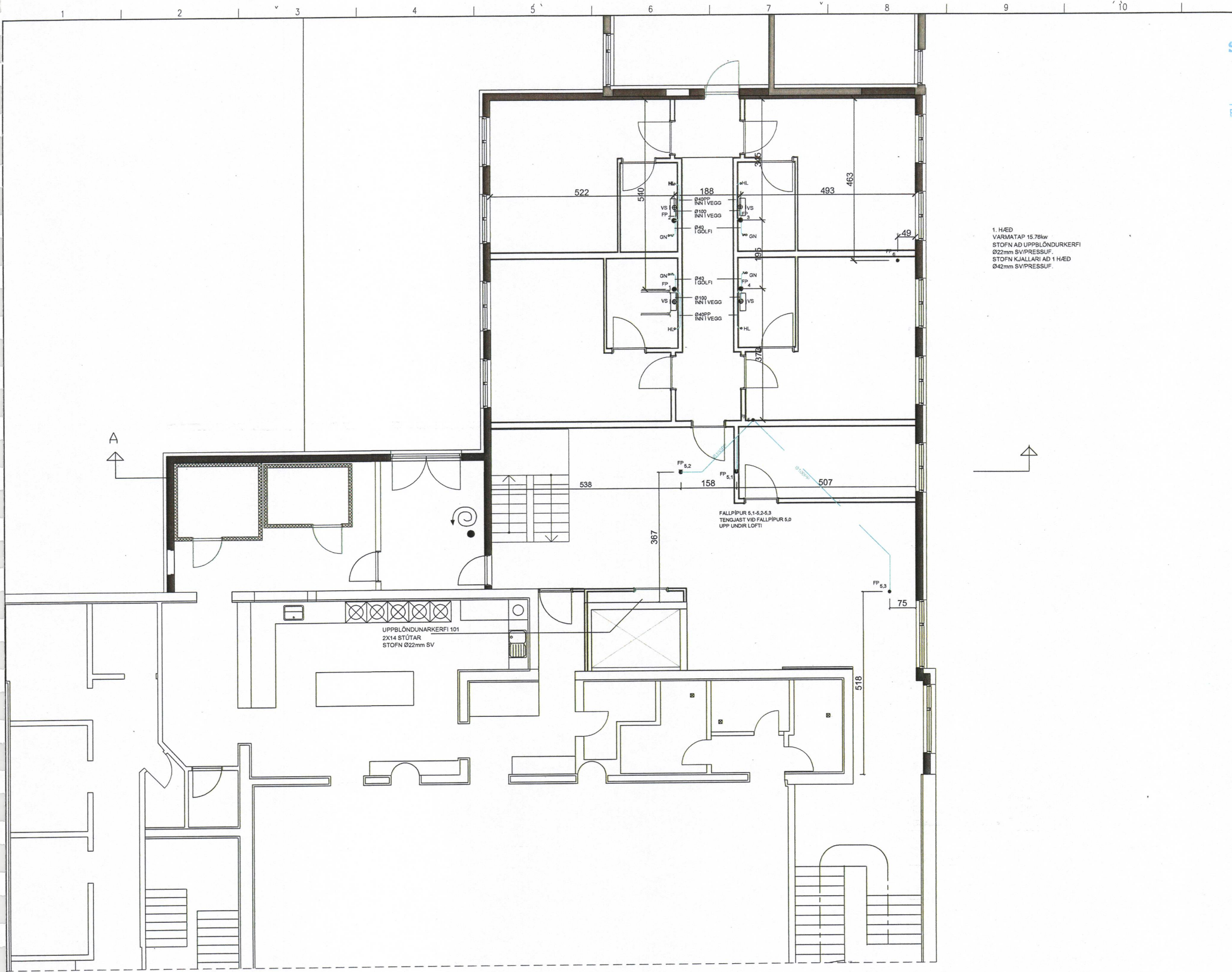
GRUNNMYND 2. HÆÐ FRÁRENNSLI M=1:50
