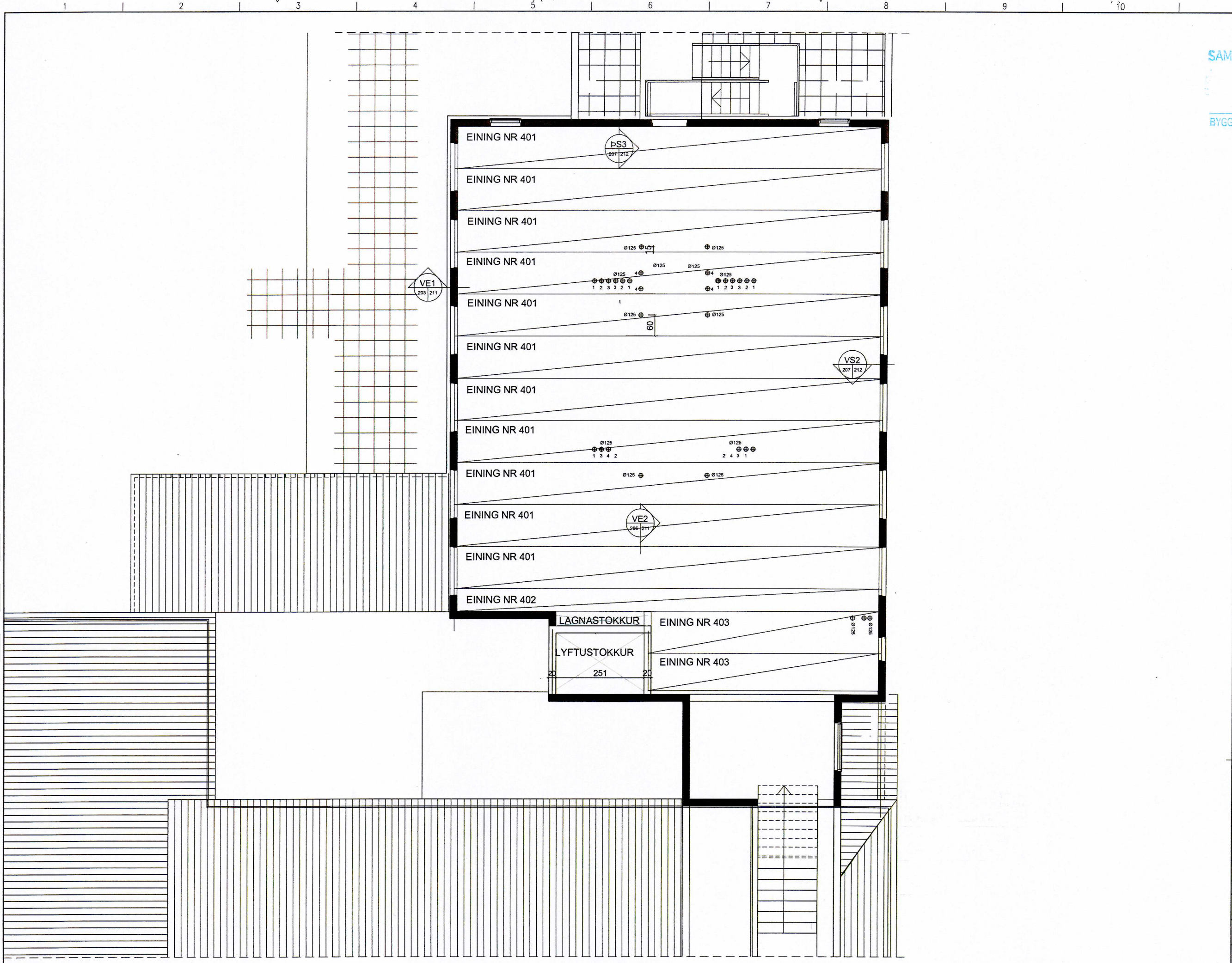
GRUNNMYND PLÖTUR YFIR 4. HÆÐ M=1:50
