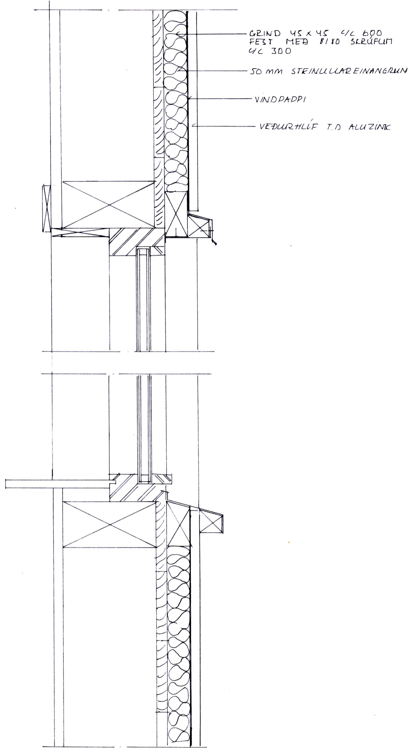
LÓDRÉTT SNÍÐ Í TRÉÚTVEGG MKV 1:5
