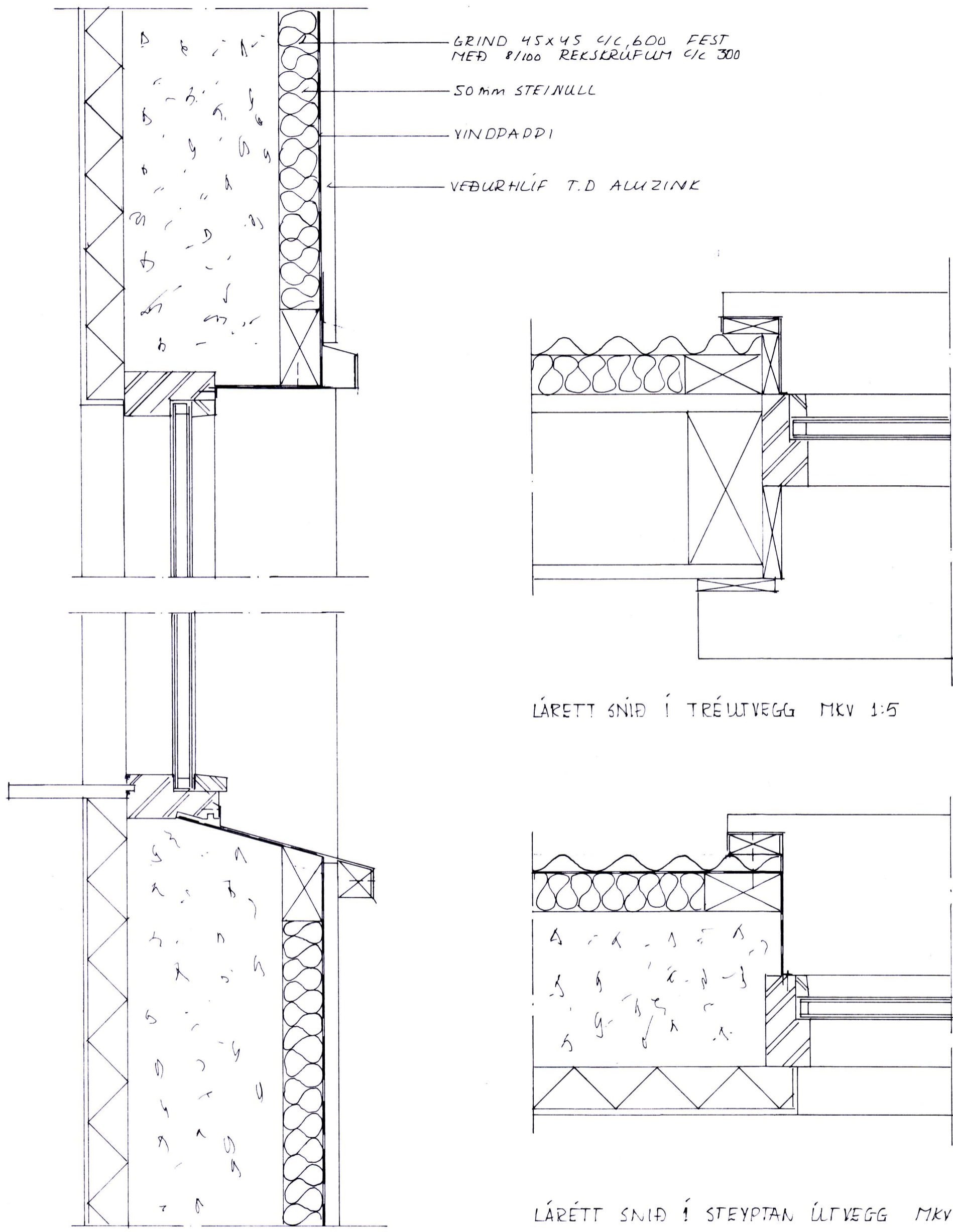
LÓDRÉTT SNÍÐ Í STEYPTAN VEGG MKV 1:5
