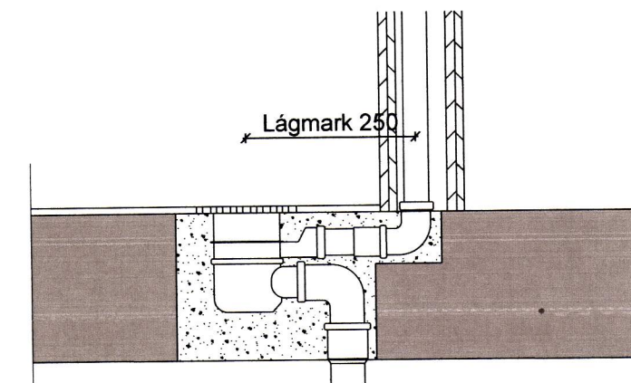
GÓLFNIÐURFALL MEÐ GEGNURENNSLI, MKV.:1:10
