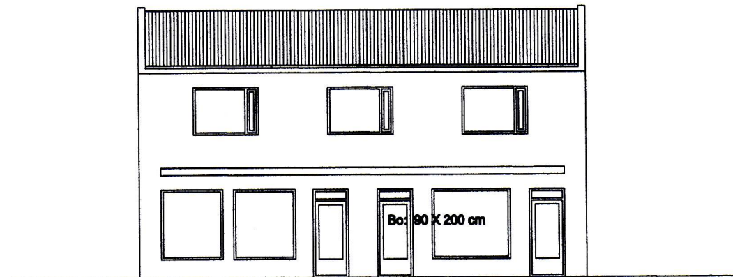
Útlit suður 1:100
