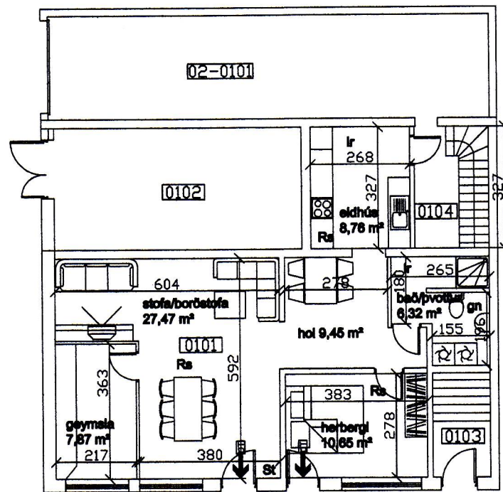
Grunnmynd 1:100
