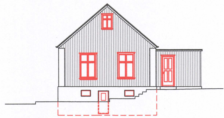
vestur
