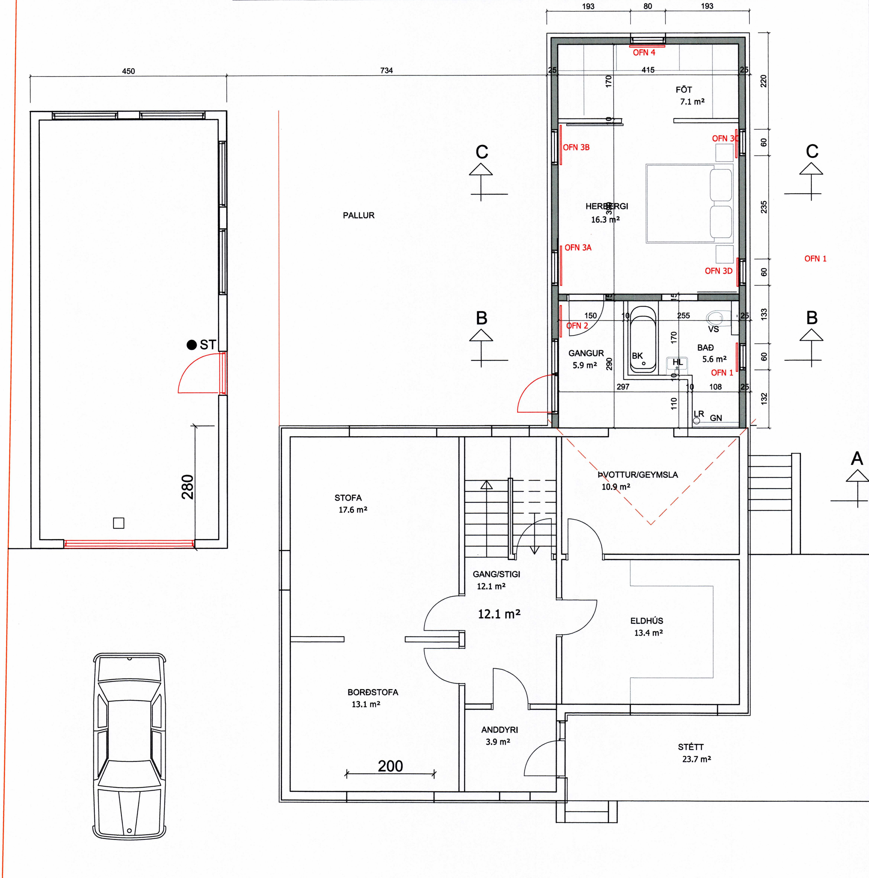
GUNNMYND 1.HÆÐ 1:50
