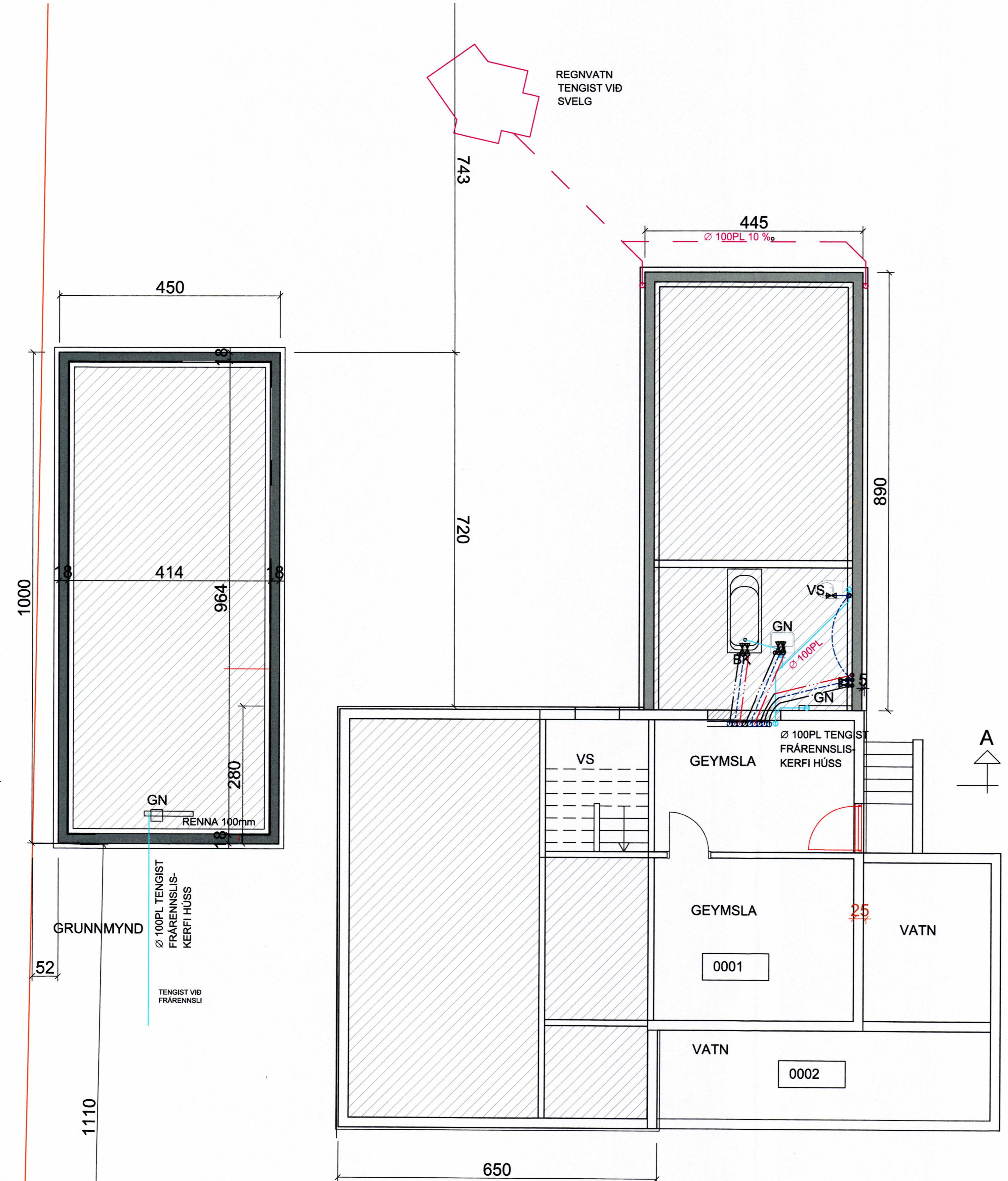
GRUNNMYND KJALLARI
