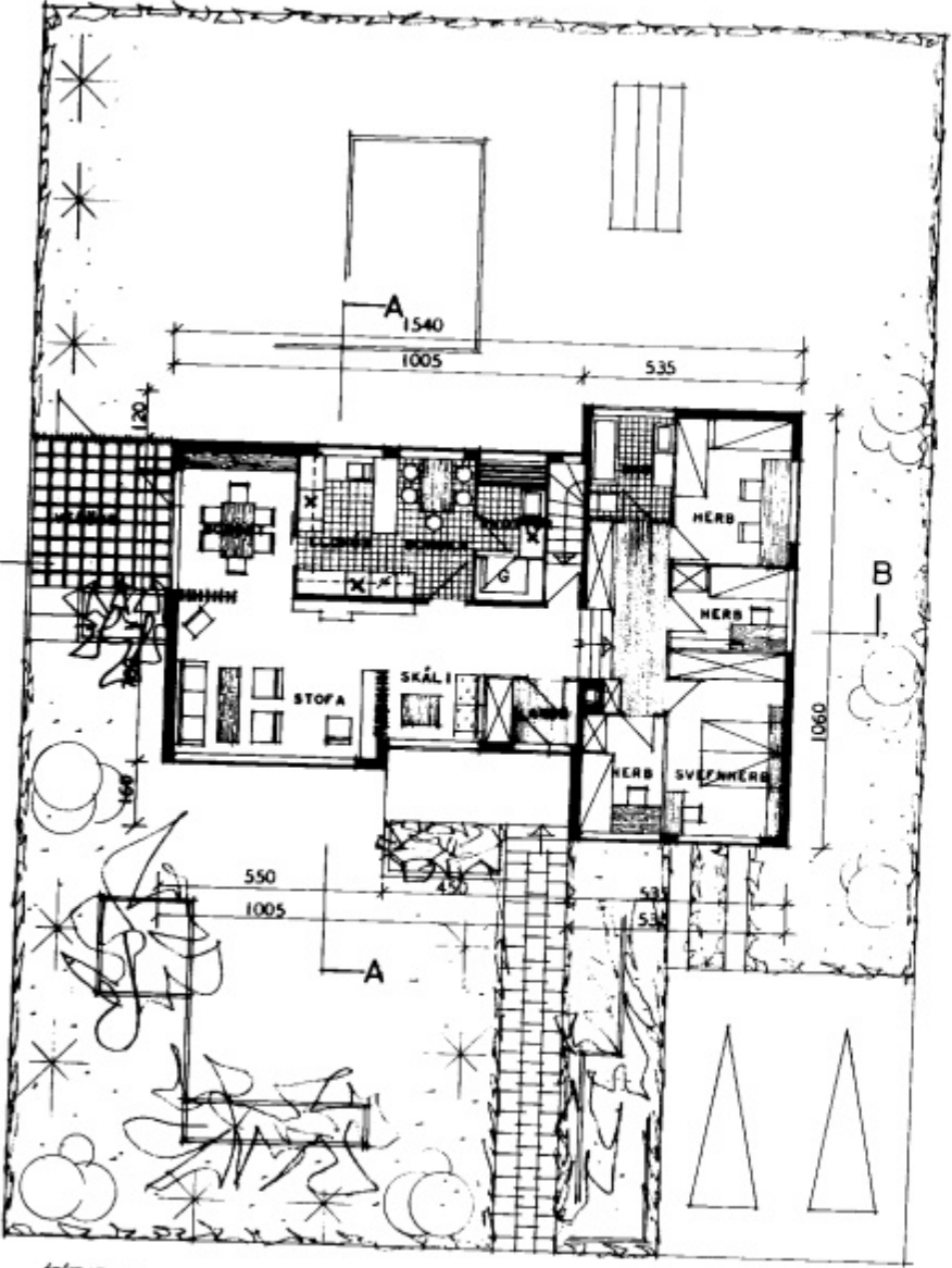
ÍBÚÐARHÆÐ
