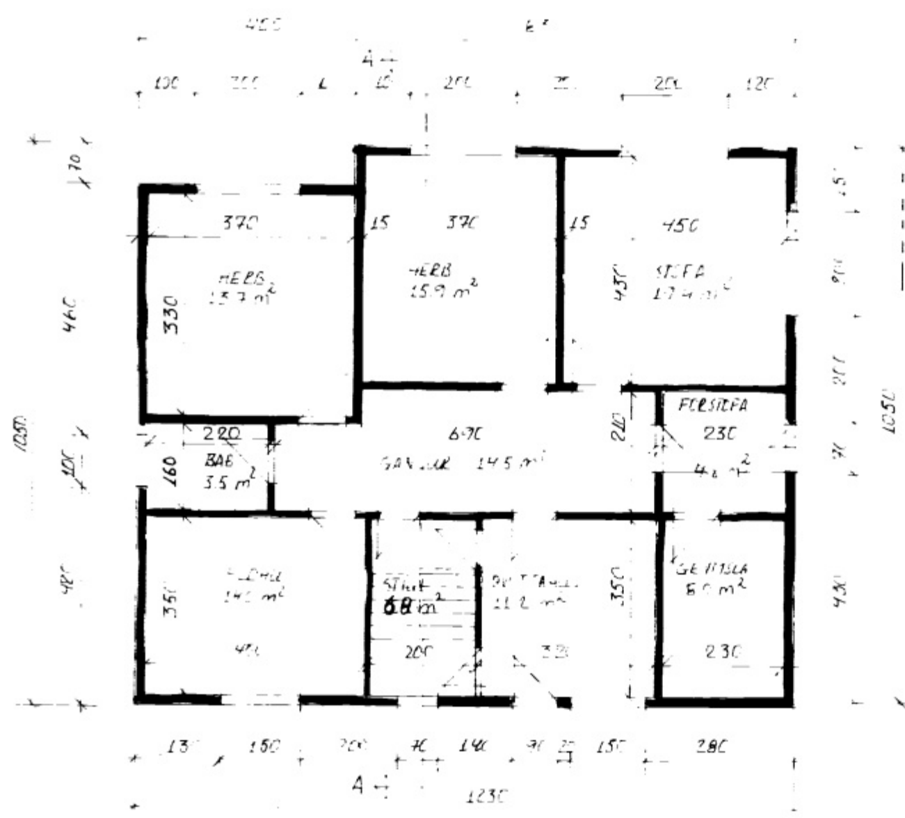
GRUNNMUND 1 HAF MKV 1:100
