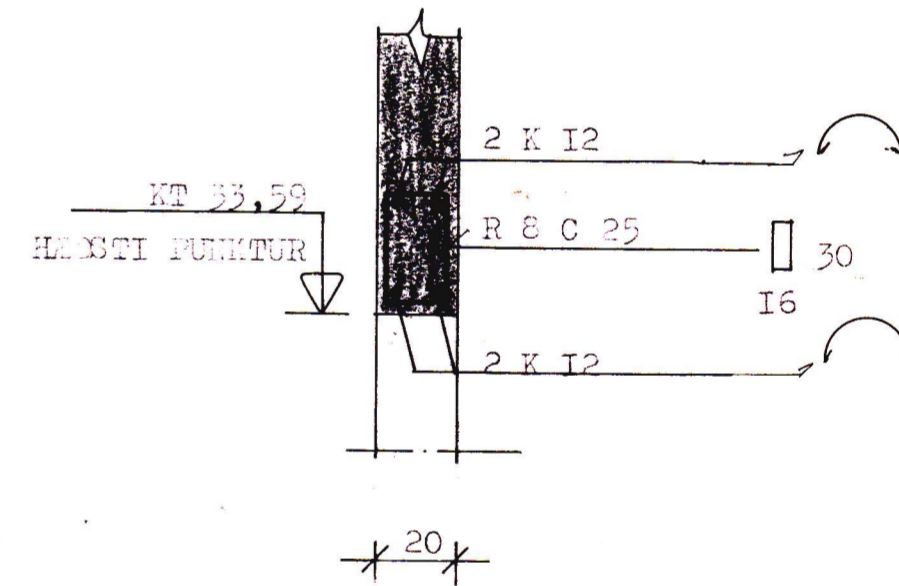
SNID L - L. I:20.
