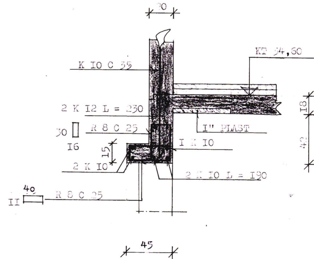
SNID K - K. I:20.
