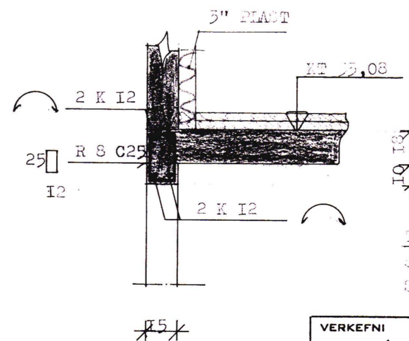
SNID K - K. I:20.
