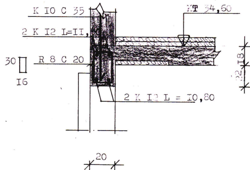
SNID J - J. I:20.
