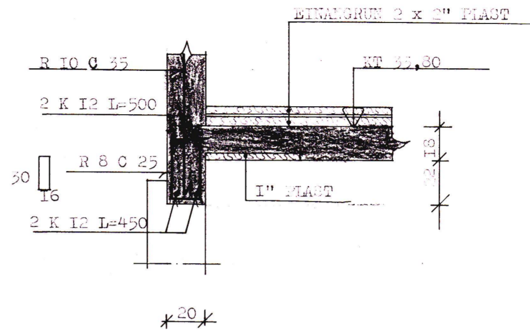
SNID G - G. I:20.
