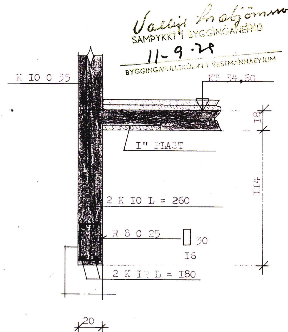
SNID H - H. I:20.
