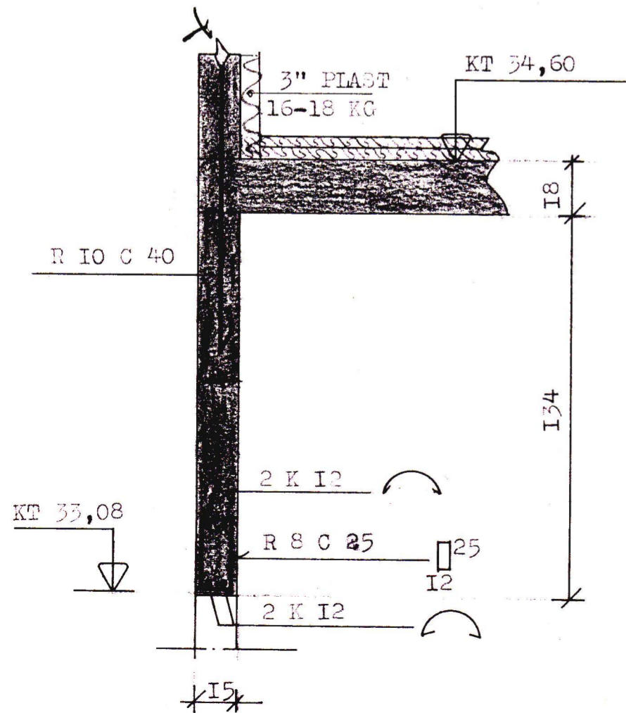
SNID I - I. I:20.
