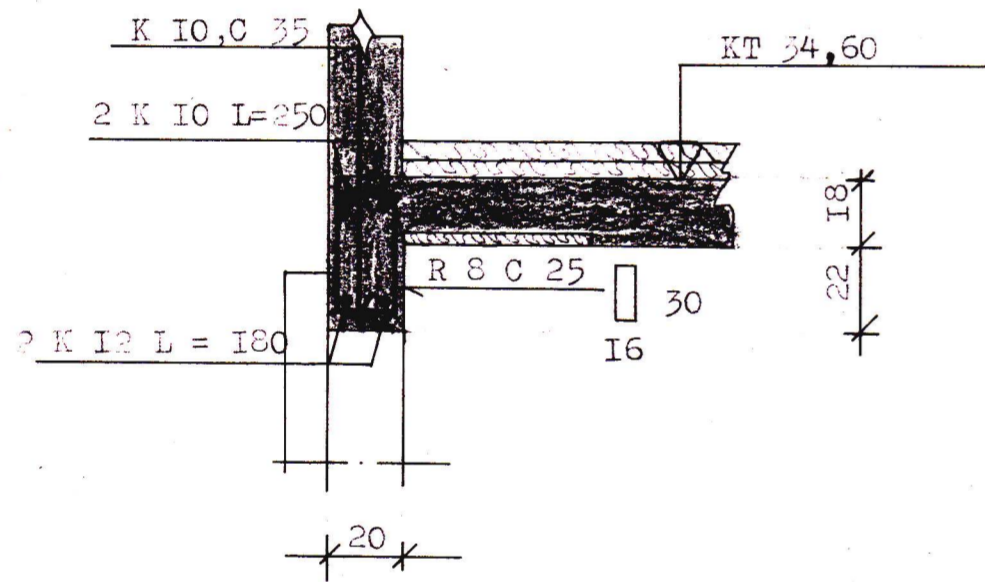
SNID I - I. I:20.
