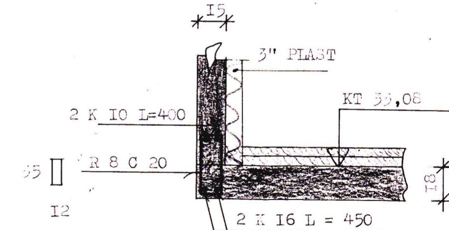
SNID L - L. I:20.
