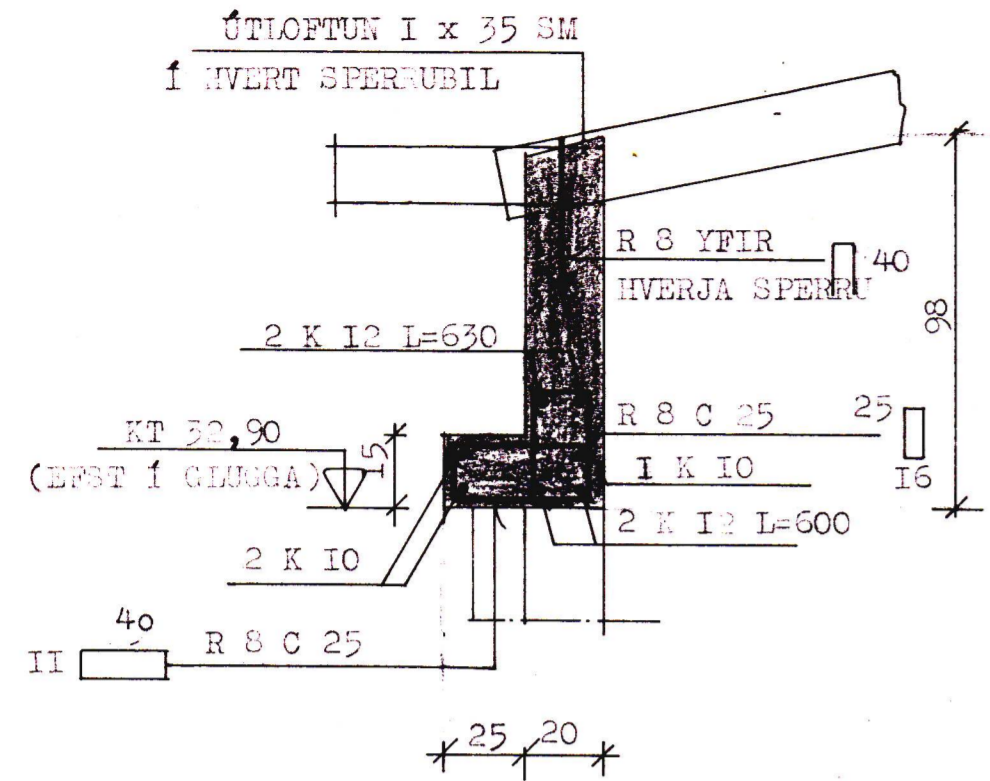
SNID E - E. I:20.
