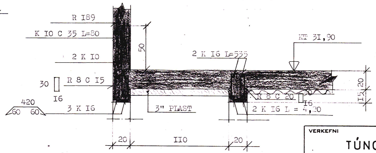
SNID J - J. I:20.
