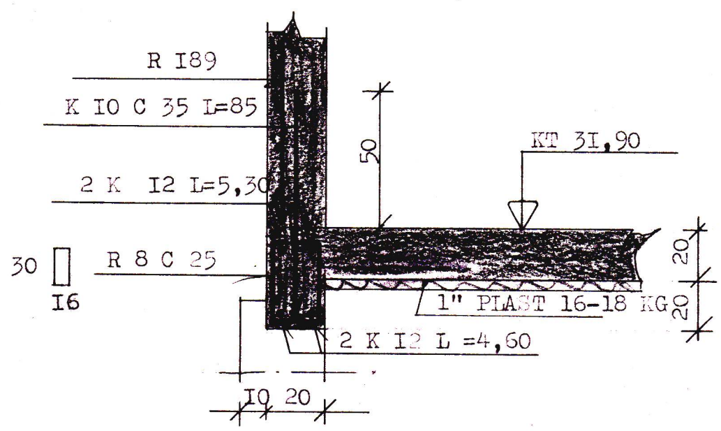
SNID I - I. I:20.
