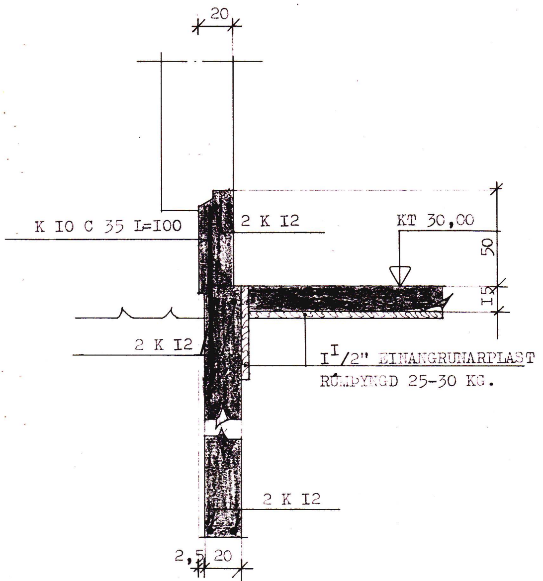
SNID A - A. I:20.
