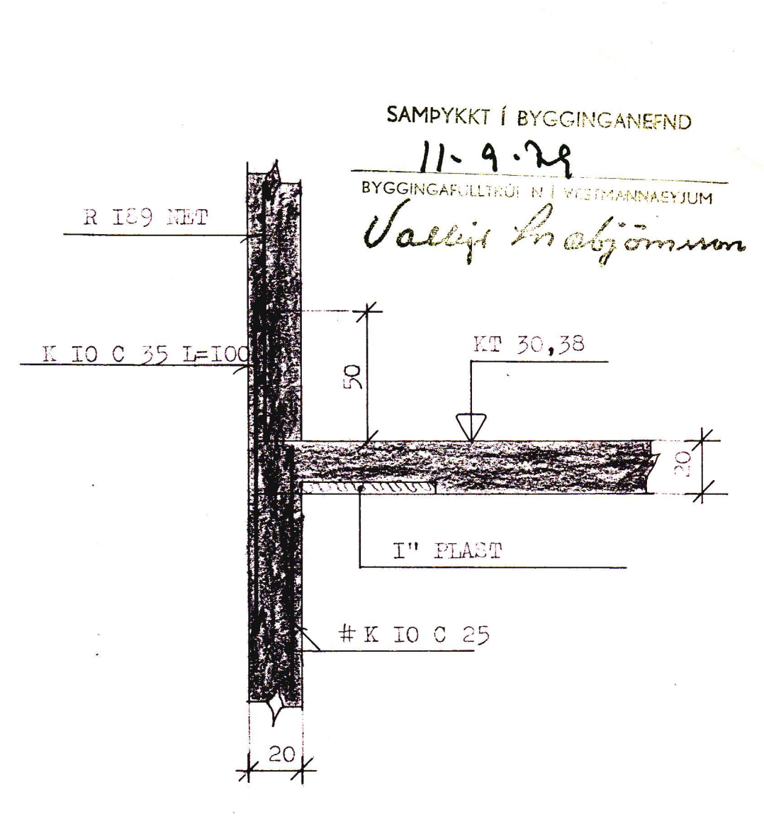
SNID D - D. I:20.
