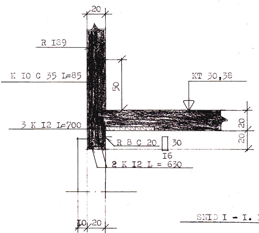
SNID E - E. I:20.
