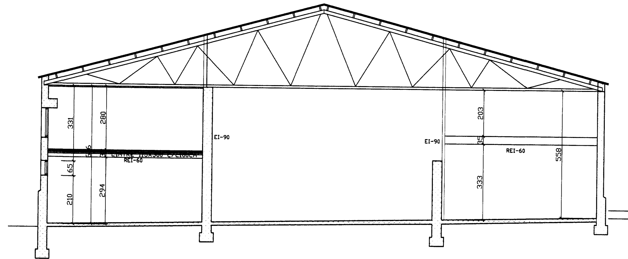
ÞVERSNID M=1:100
