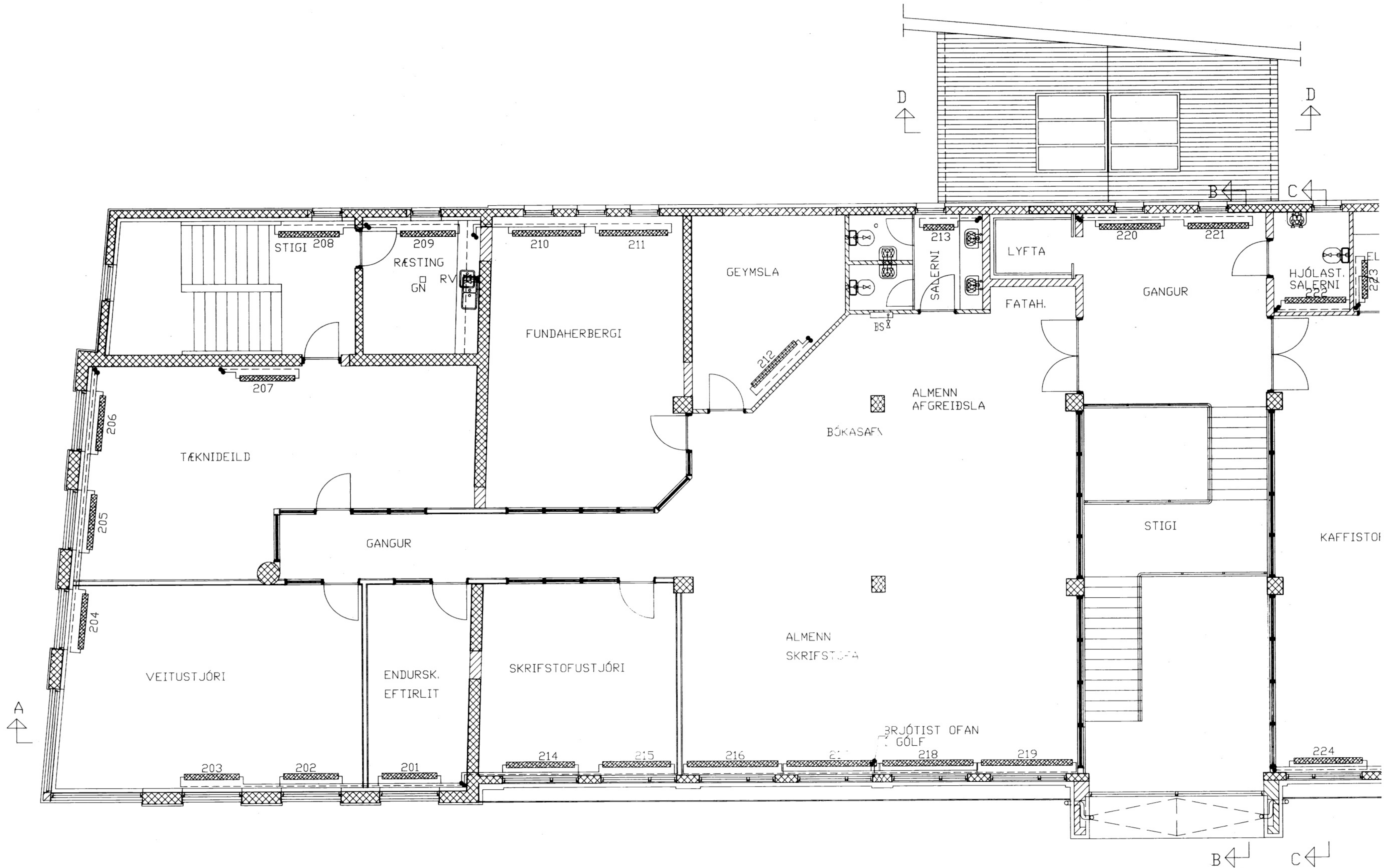
GRUNNMYND 2.HÆÐ M=1:100
