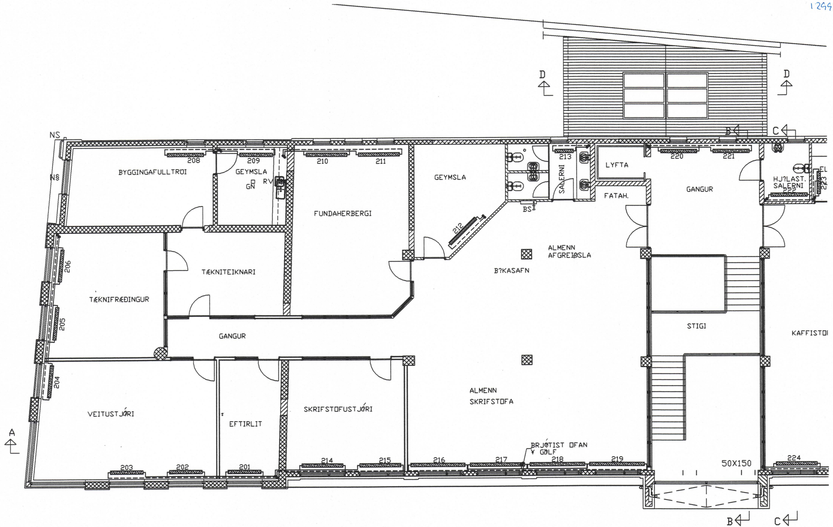
GRUNNMYND 2.HÆÐ=1:100
