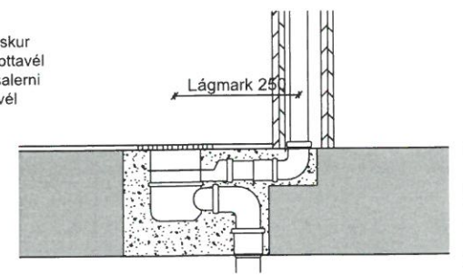
GÓLFNIÐURFALL MED GEGNURENNSLI, MKV.:1:10
