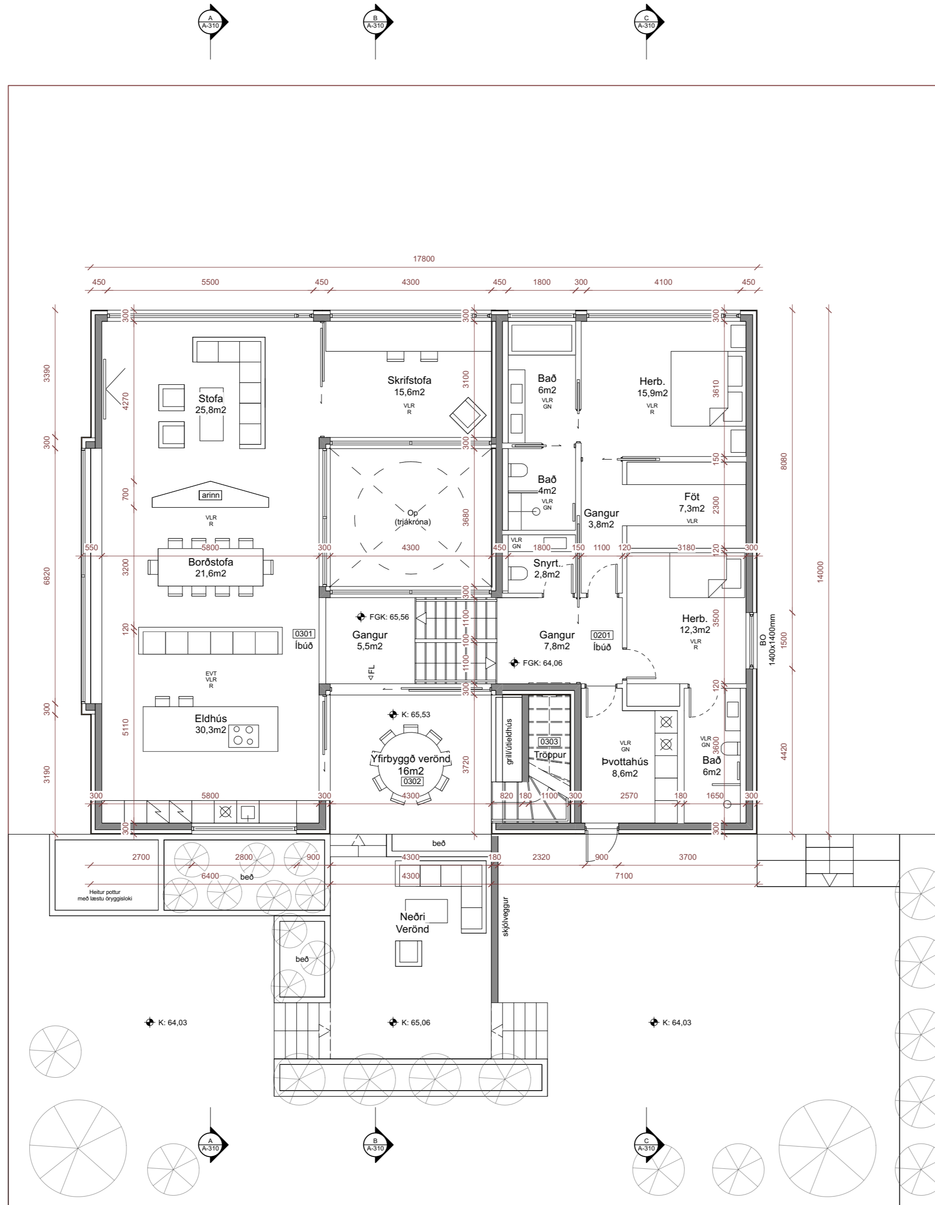
Grunnmynd efri hæða mkv: 1:100
